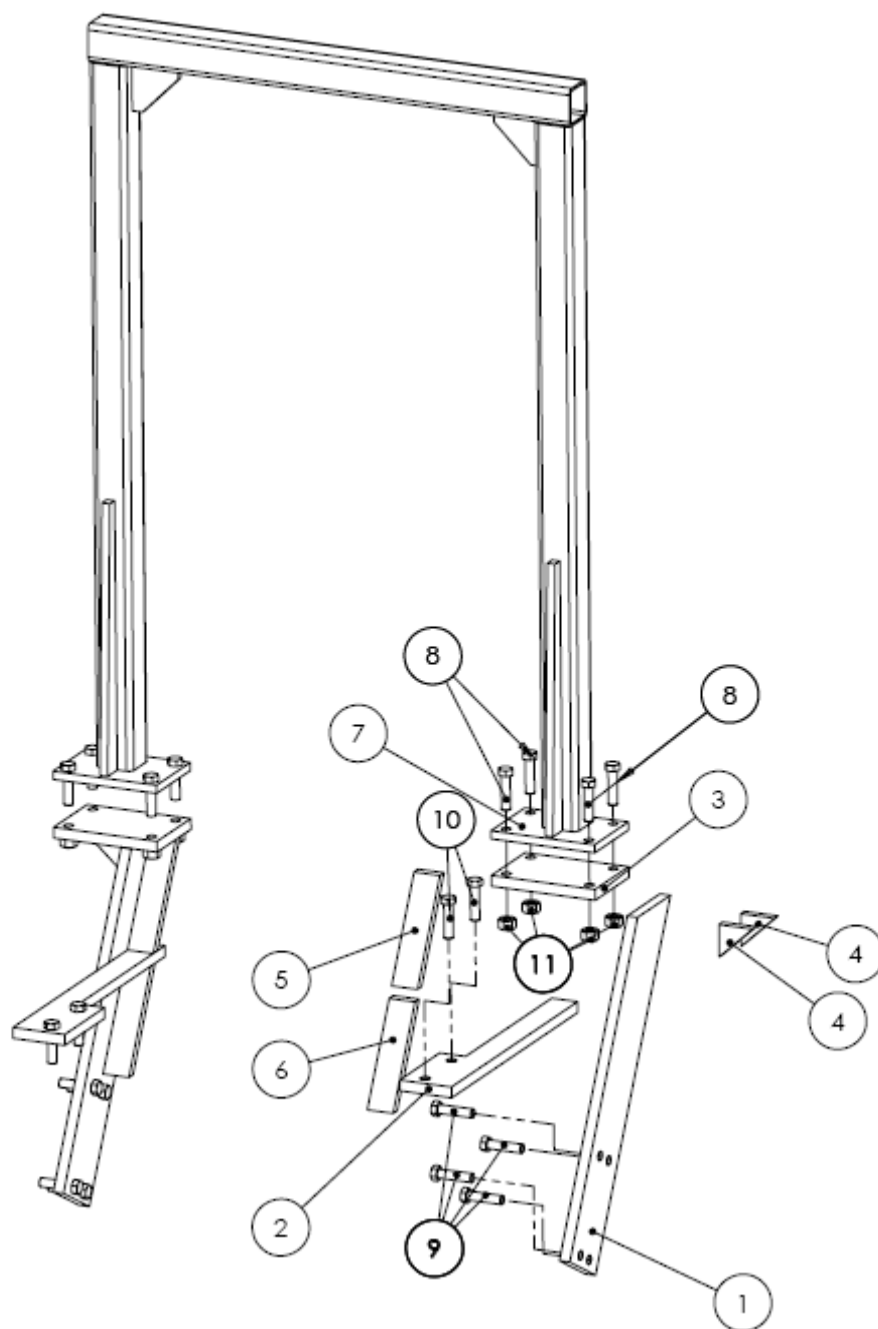
Figura 1. Struttura di protezione contro il rischio di ribaltamento a due montanti posteriori per trattori a cingoli modello Landini 6500C e simili
