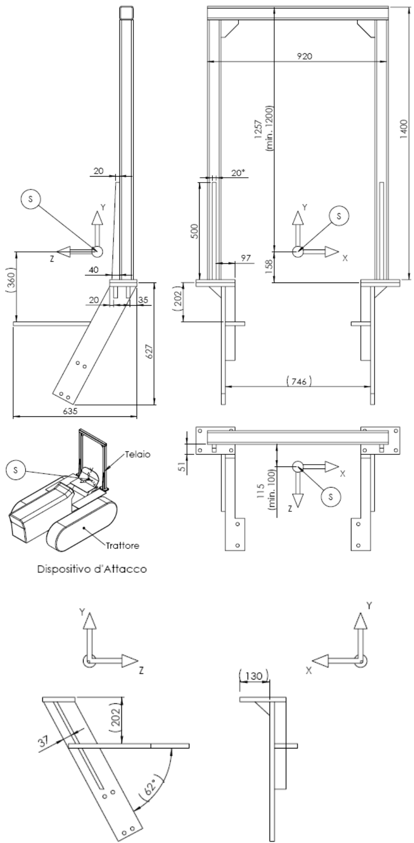
Figura 2. Quote di assemblaggio
