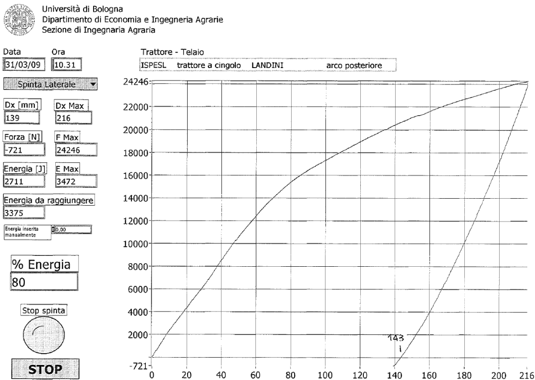
Figura 11. Spinta laterale destra
