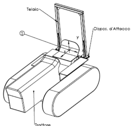
Figura 10. Struttura di protezione per trattori a cingoli modello Landini 6500C e simili
