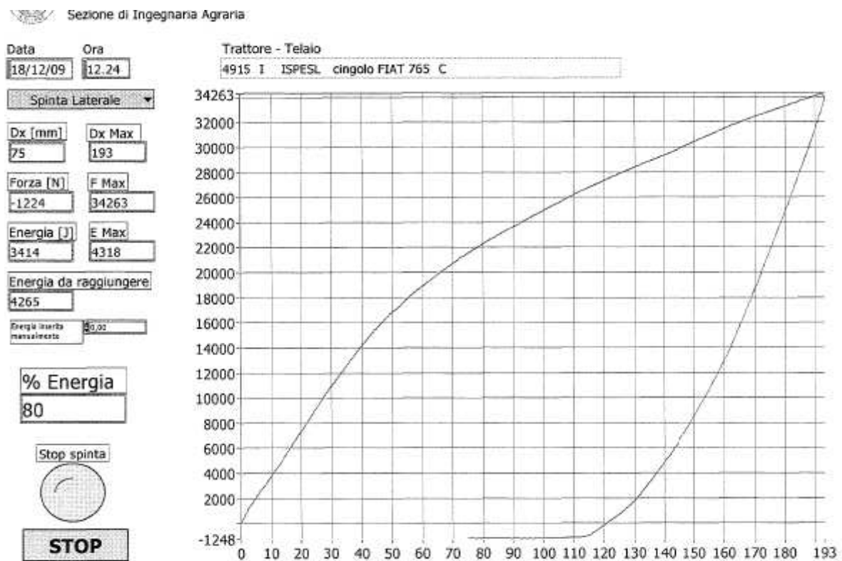
Figura 14. Spinta laterale destra
