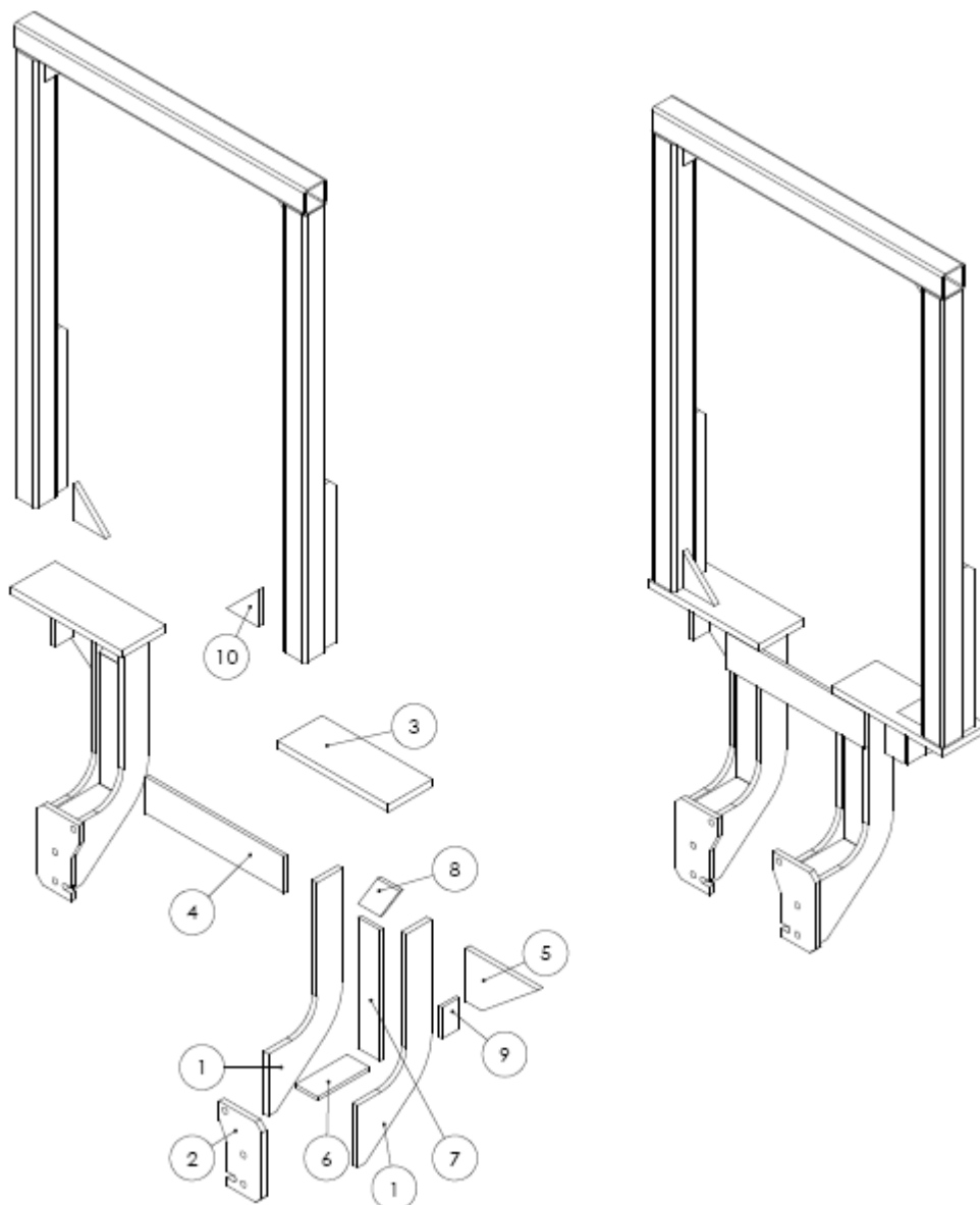
Figura 1. Struttura di protezione contro il rischio di ribaltamento a due montanti posteriori per trattori a cingoli modello Fiat 765 C e simili (Fiat 665 CM)
