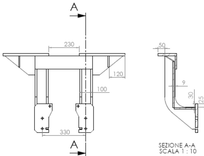
Figura 2. Quote di assemblaggio
