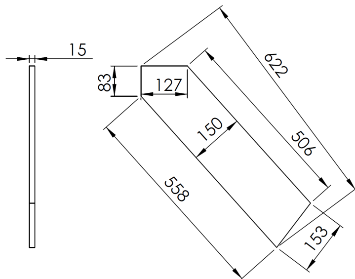
Figura 4. Elemento A2
