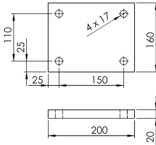
Figura 5. Elemento A3
