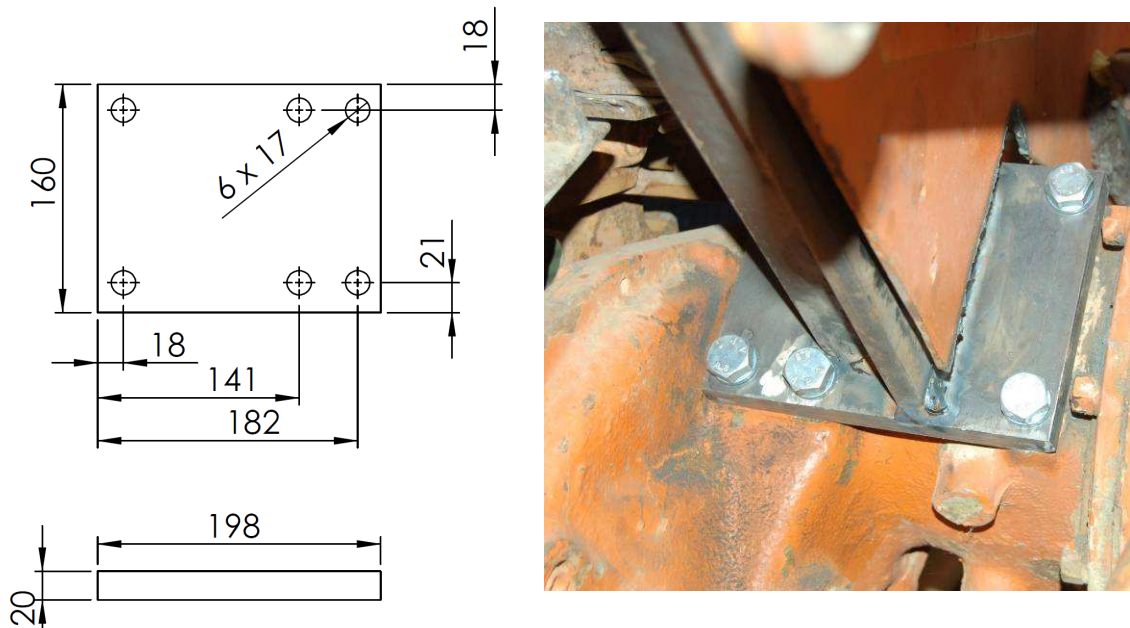
Figura 3. Elemento A1
