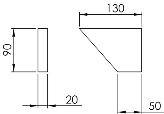
Figura 8. Elemento A6
