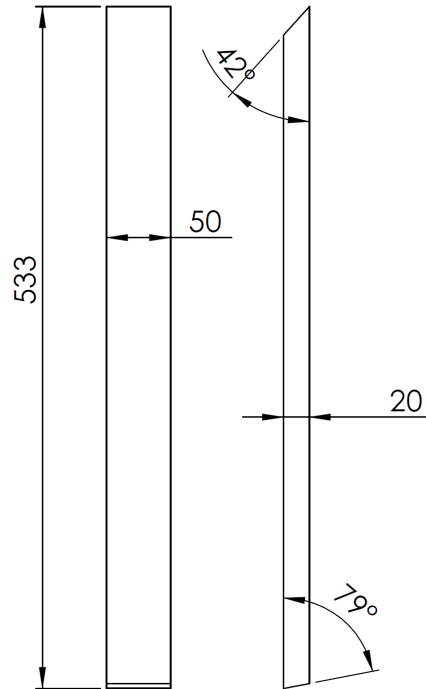
Figura 7. Elemento A5
