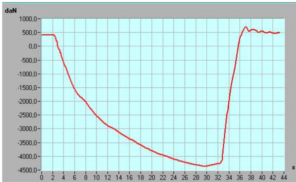
Figura 11. Schiacciamento
