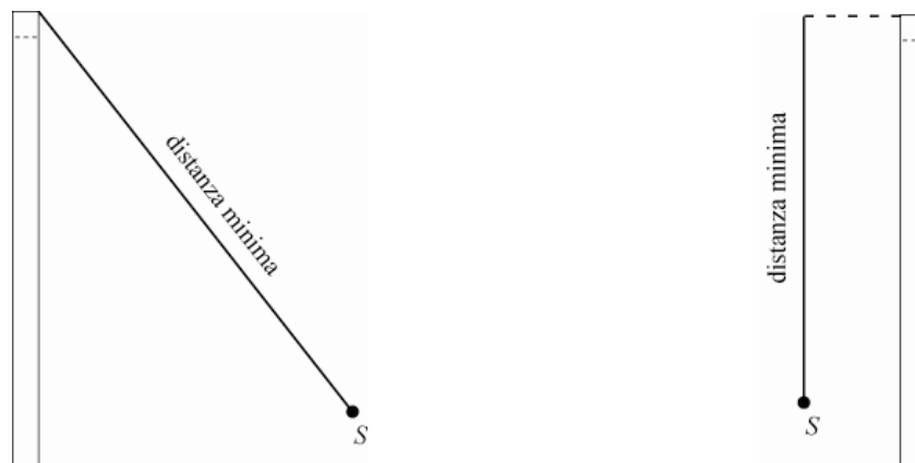
Figura 8 – Distanza minima per motoagricole rese conformi con telaio di protezione rispondente ai requisiti previsti dalla sezione 1 del presente documento
