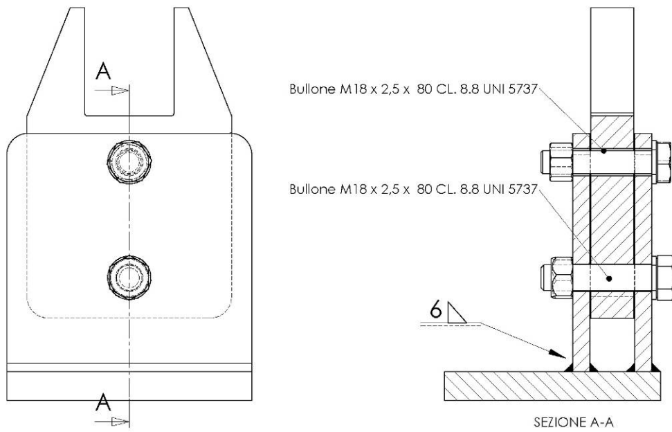
Figura 5. Assieme dell'elemento di collegamento per telaio fisso
