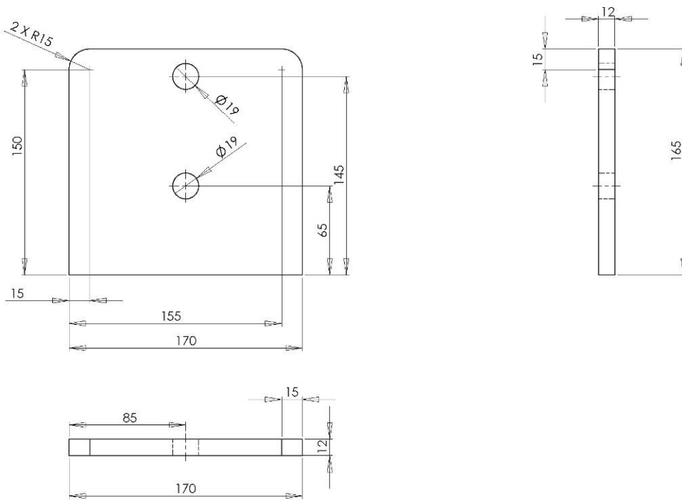
Figura 4. Piastra laterale per telaio fisso
