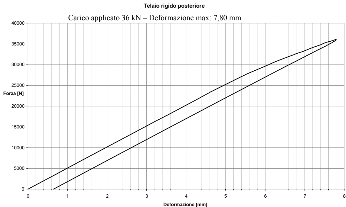
Figura 17. Telaio rigido posteriore: diagramma Forza vs. Deformazione
