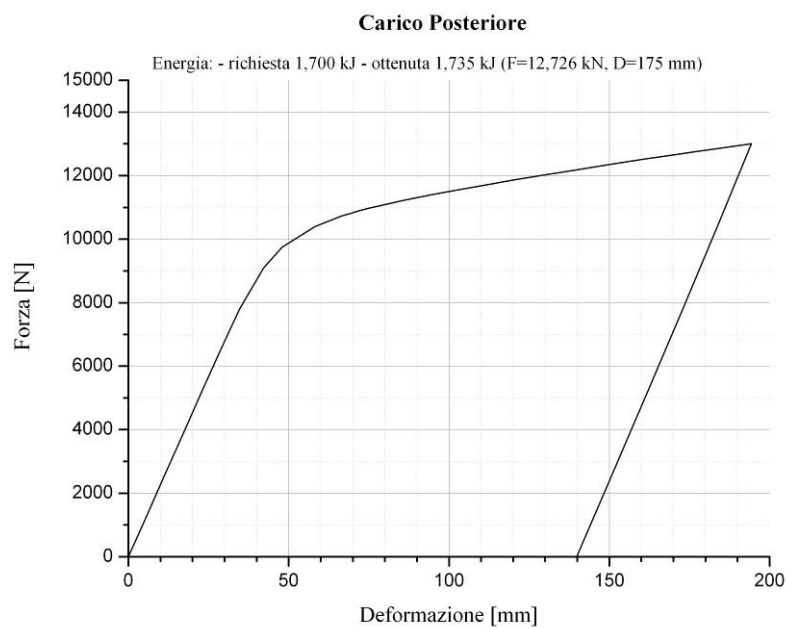
Figura 10. Carico posteriore: diagramma Forza vs. Deformazione
