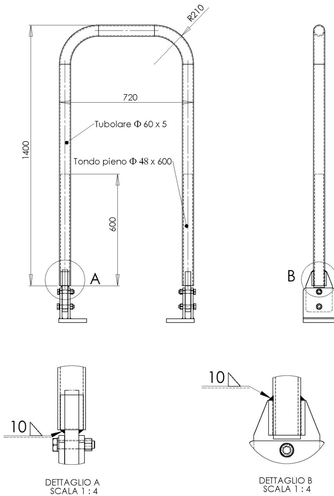
Figura 2. Telaio di protezione anteriore fisso
