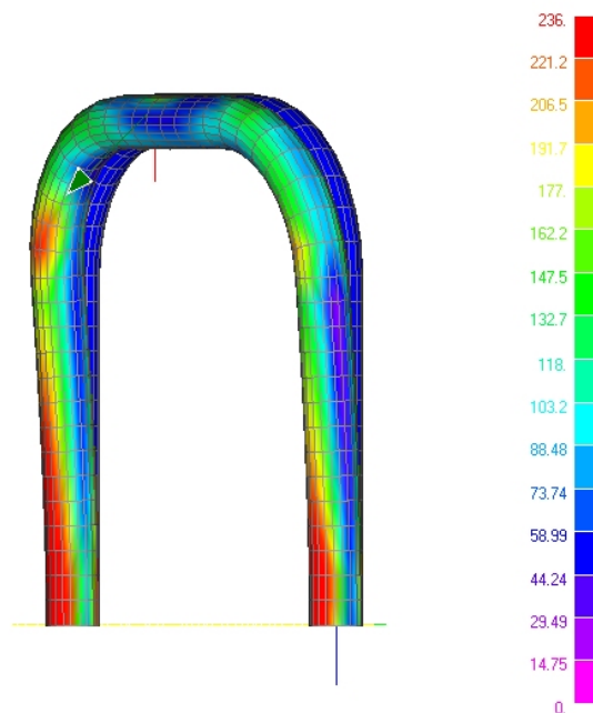
Figura 16. Telaio rigido posteriore: diagramma a falsi colori della tensione [MPa]
