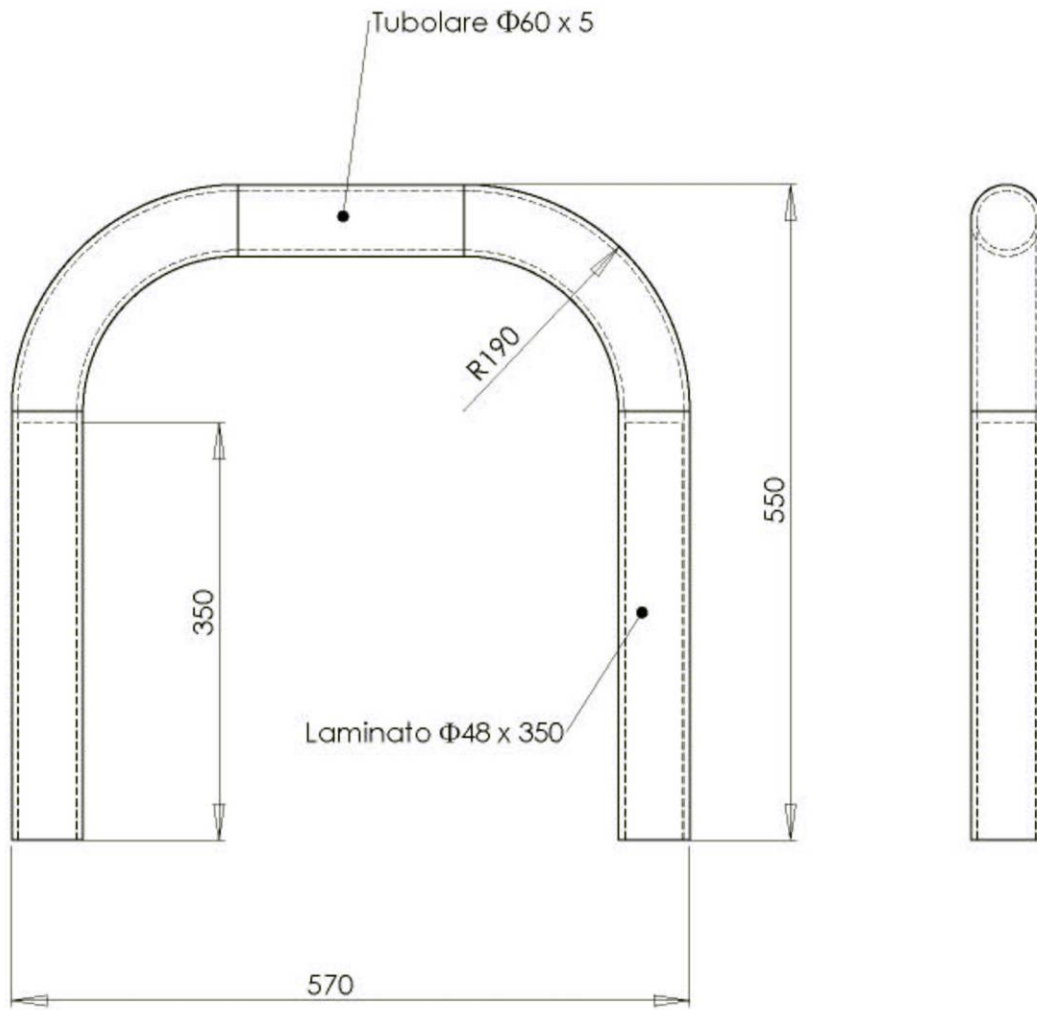
Figura 1. Telaio rigido posteriore
