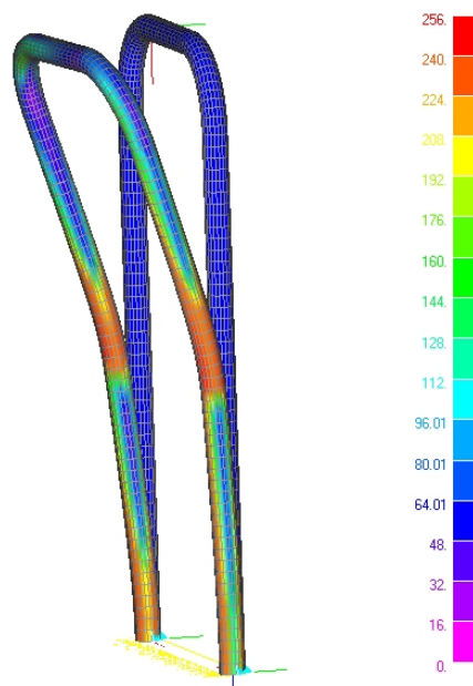
Figura 9. Carico posteriore: diagramma a falsi colori della tensione [MPa]
