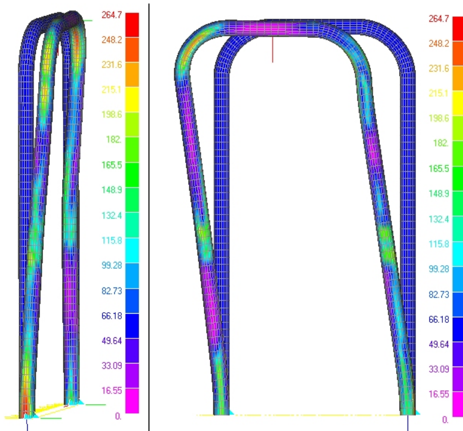
Figura 15. Deformazione residua: diagramma a falsi colori della tensione [MPa]
