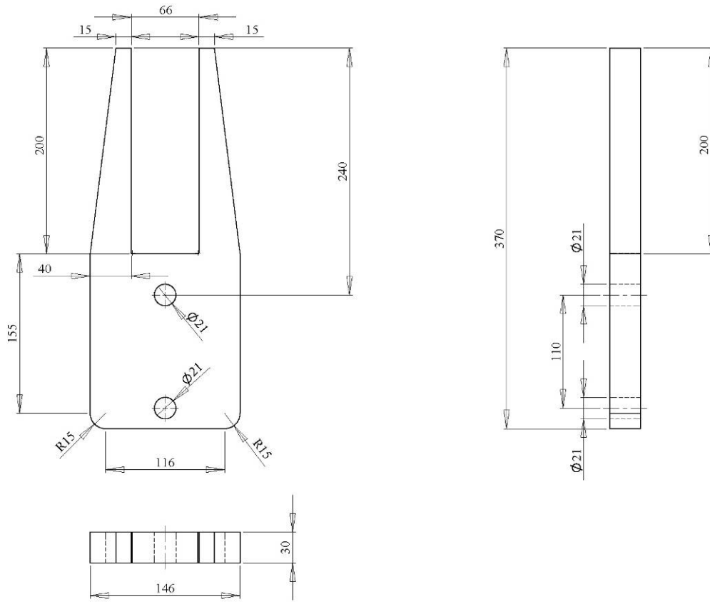
Figura 3. Piastra interna di collegamento per telaio fisso
