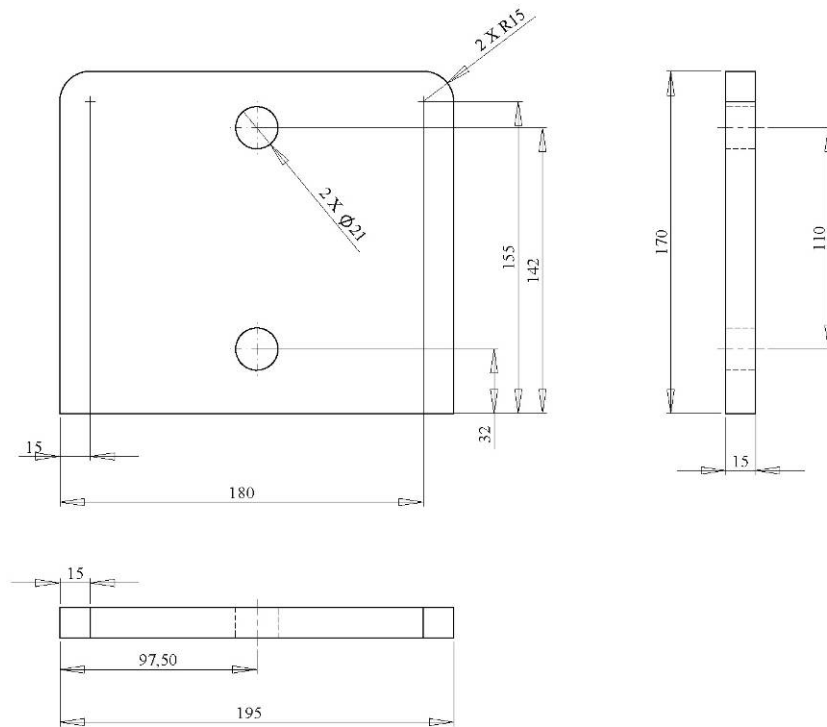
Figura 4. Piastra laterale interna per telaio fisso
