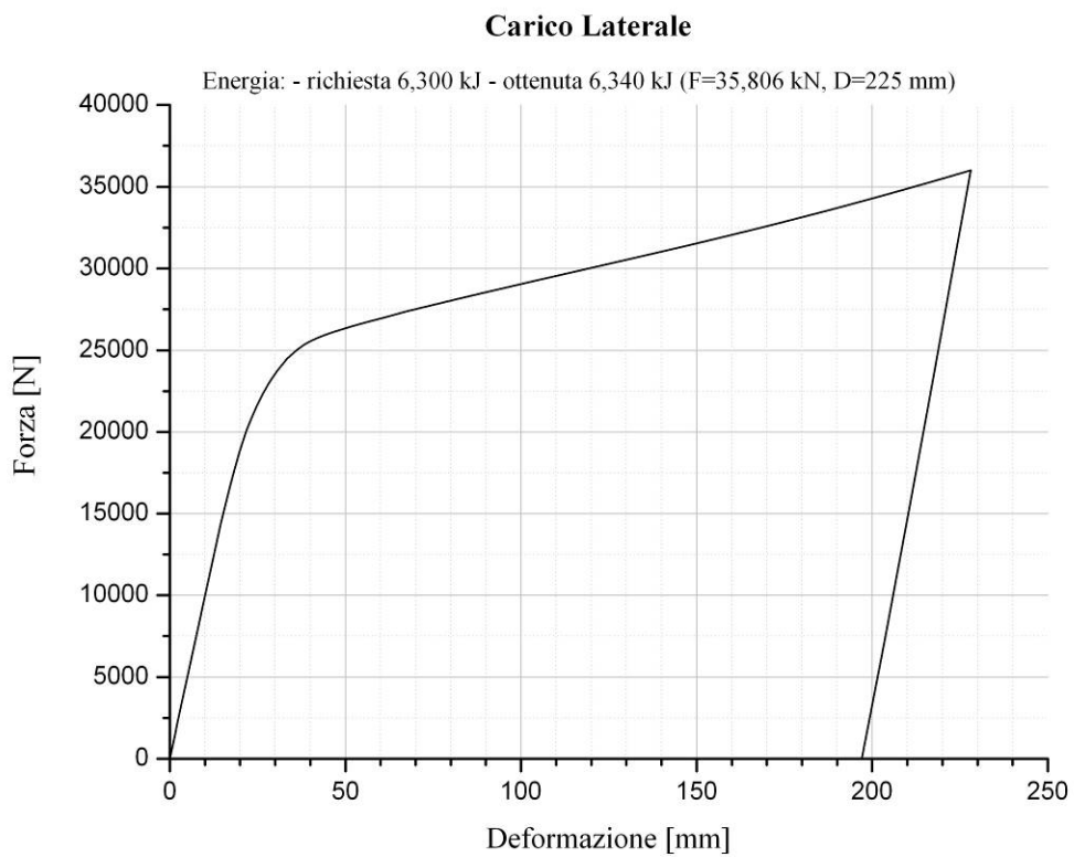
Figura 14. Carico laterale: diagramma Forza vs. Deformazione
