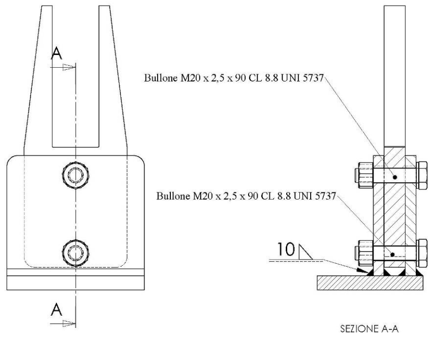
Figura 5. Assieme dell'elemento di collegamento per telaio fisso
