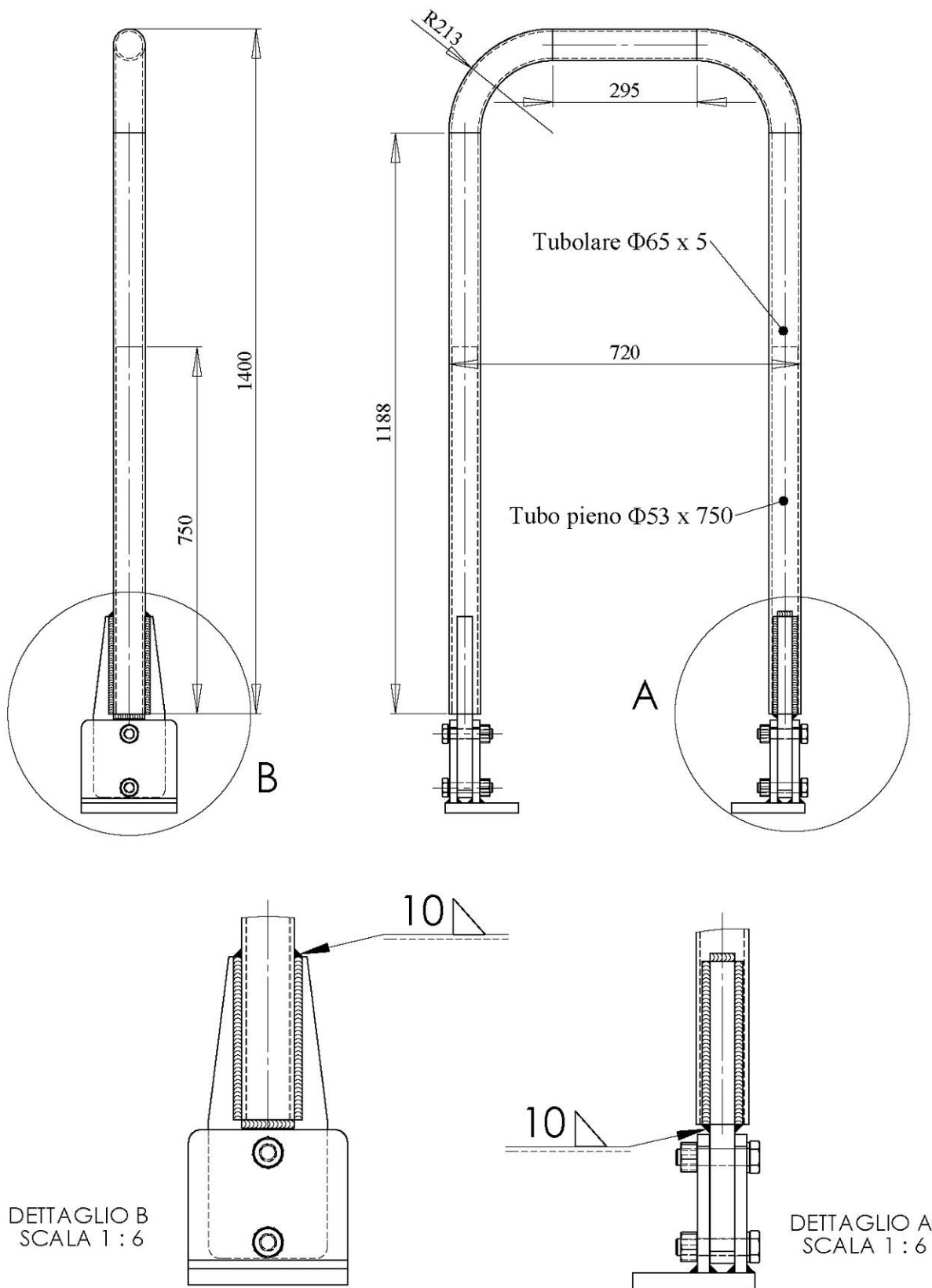
Figura 2. Telaio di protezione anteriore fisso
