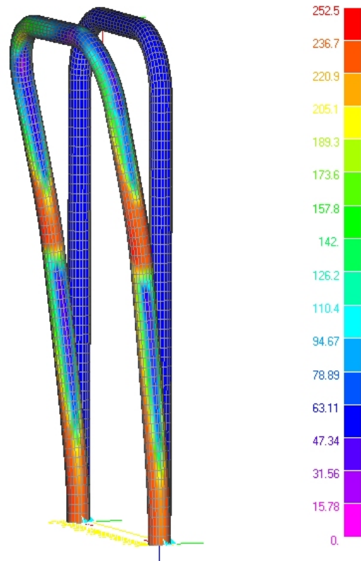
Figura 9. Carico posteriore: diagramma a falsi colori della tensione [MPa]
