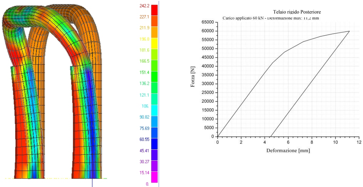
Figura 16. Telaio rigido posteriore: diagramma a falsi colori della tensione [MPa] e diagramma Forza vs. Deformazione
