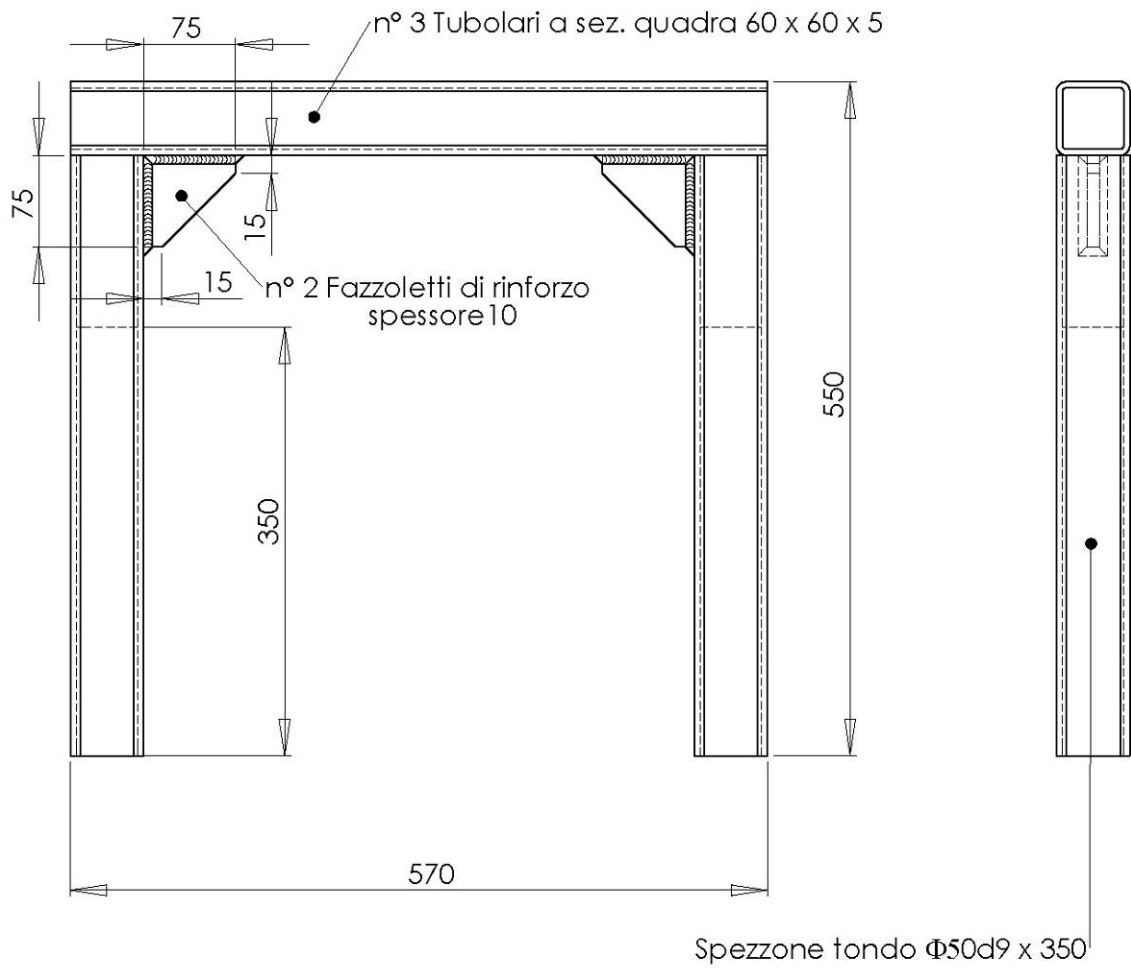
Figura 1. Telaio rigido posteriore
