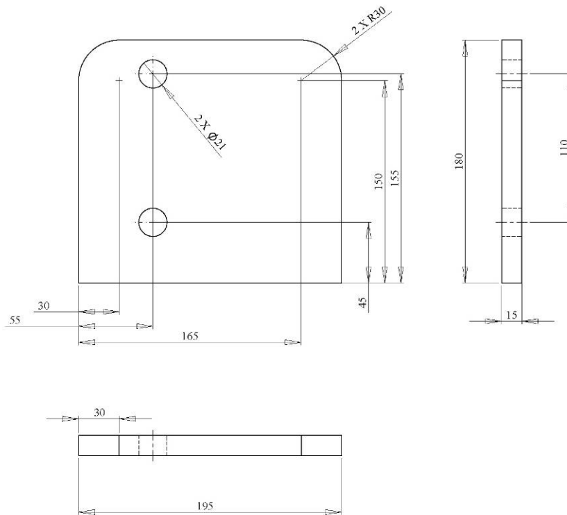
Figura 4. Piastra laterale interna per telaio abbattibile
