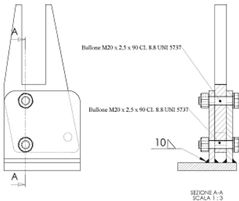
Figura 5. Assieme dell'elemento di collegamento per telaio abbattibile
