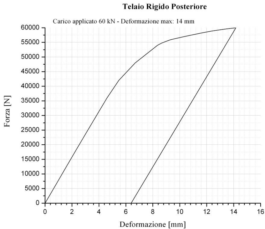
Figura 17. Telaio rigido posteriore: diagramma Forza vs. Deformazione
