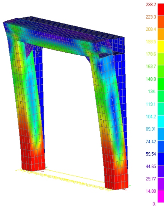
Figura 16. Telaio rigido posteriore: diagramma a falsi colori della tensione [MPa]
