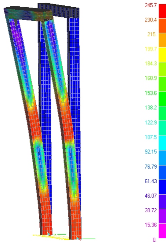
Figura 9. Carico posteriore: diagramma a falsi colori della tensione [MPa]
