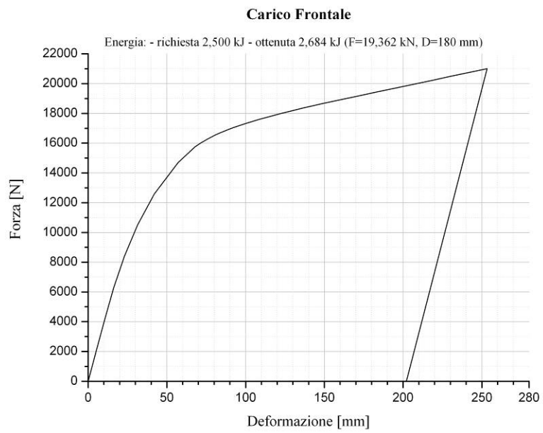
Figura 12. Carico frontale: diagramma Forza vs. Deformazione
