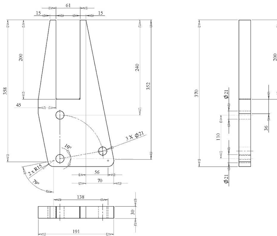
Figura 3. Piastra interna di collegamento per telaio abbattibile
