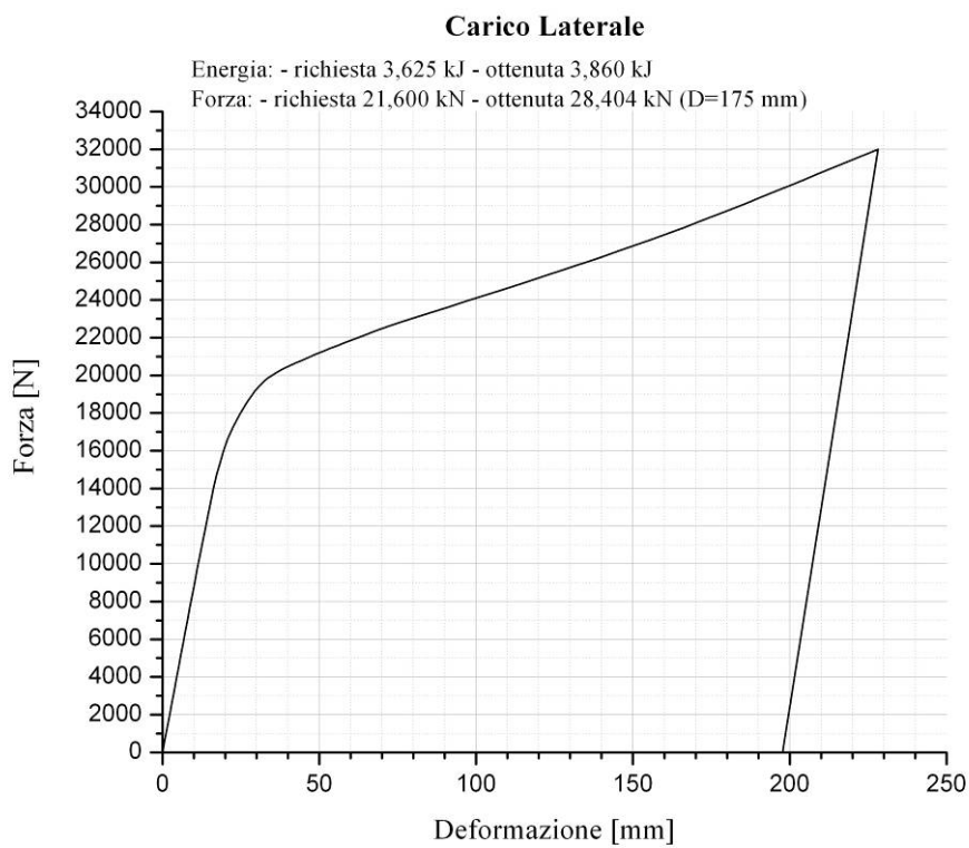
Figura 10. Carico laterale: diagramma Forza vs. Deformazione
