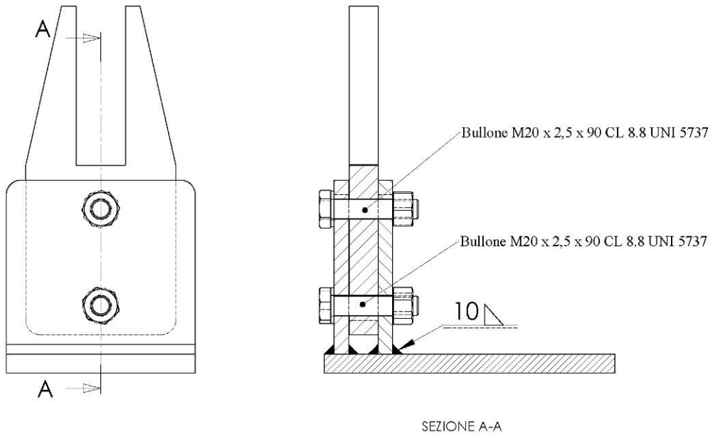
Figura 5. Assieme dell'elemento di collegamento per telaio fisso
