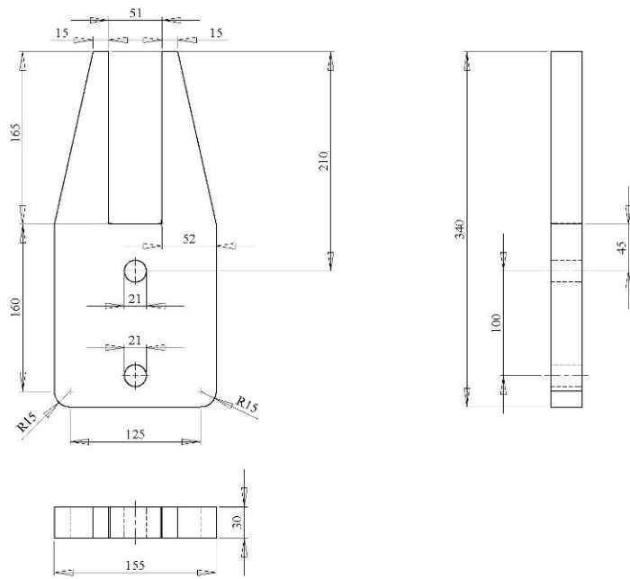
Figura 3. Piastra interna di collegamento per telaio fisso
