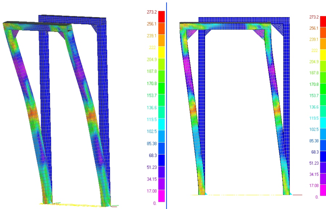
Figura 13. Deformazione residua: diagramma a falsi colori della tensione [MPa]
