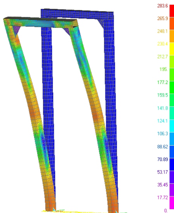
Figura 12. Carico posteriore: diagramma a falsi colori della tensione [MPa]
