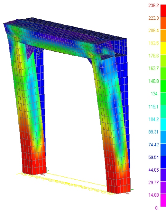
Figura 14. Telaio rigido posteriore: diagramma a falsi colori della tensione [MPa]
