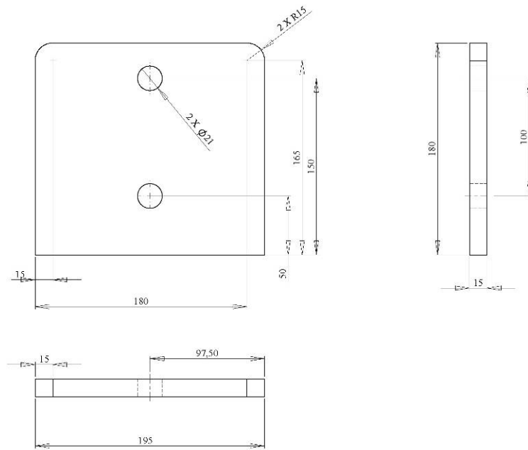
Figura 4. Piastra laterale interna per telaio fisso
