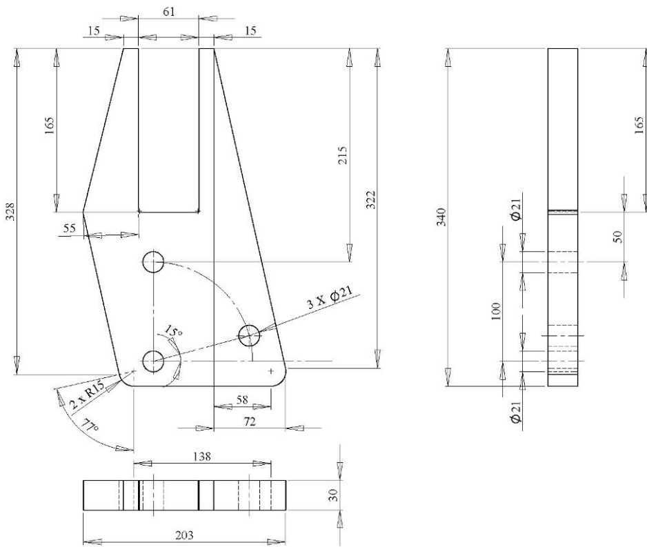
Figura 3. Piastra interna di collegamento per telaio abbattibile
