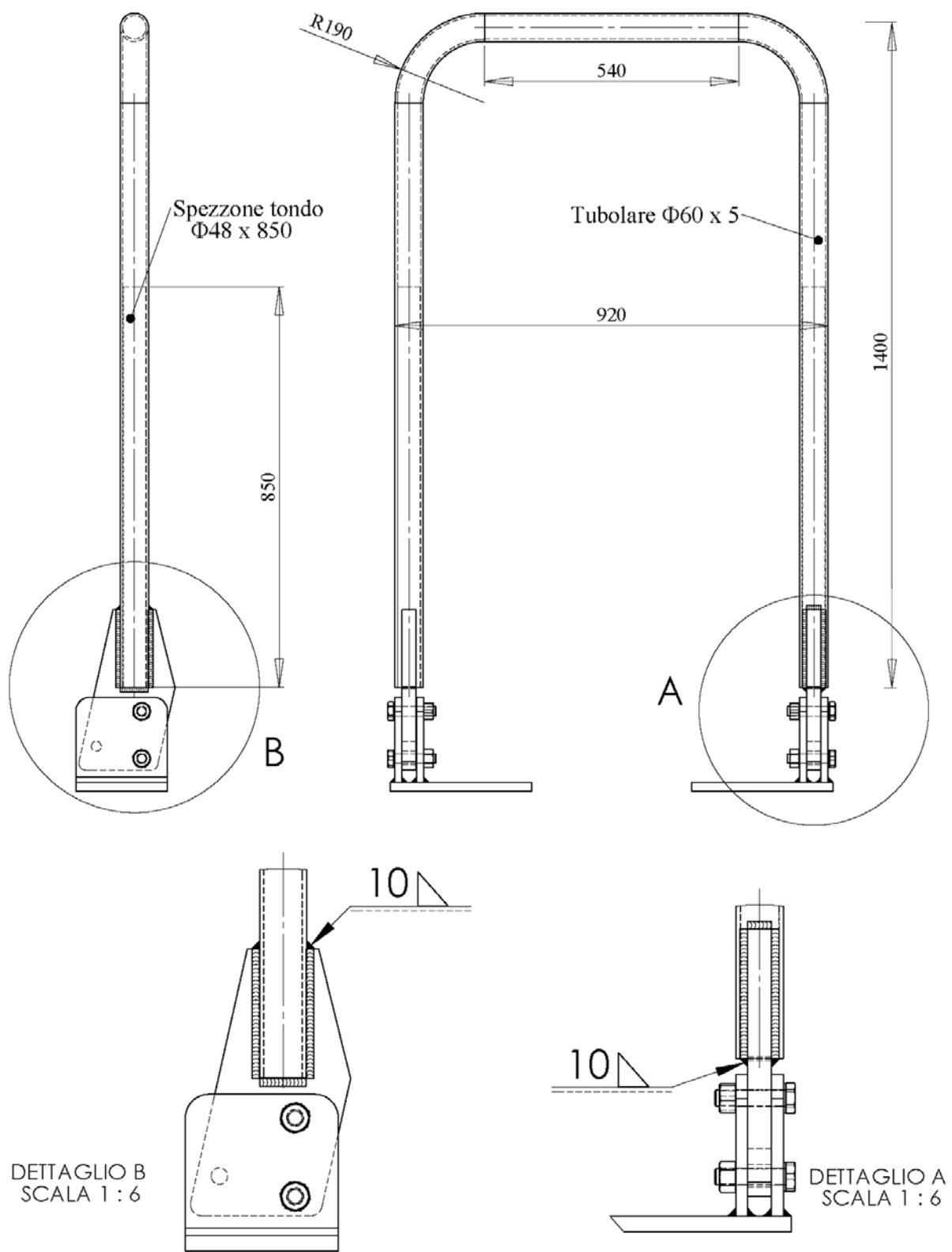
Figura 2. Telaio di protezione anteriore abbattibile
