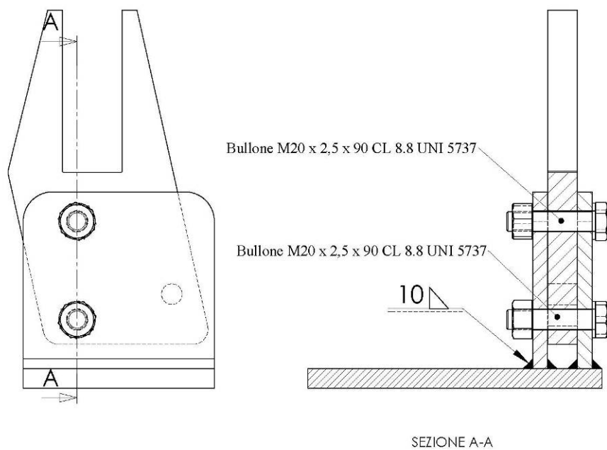
Figura 5. Assieme dell'elemento di collegamento per telaio abbattibile
