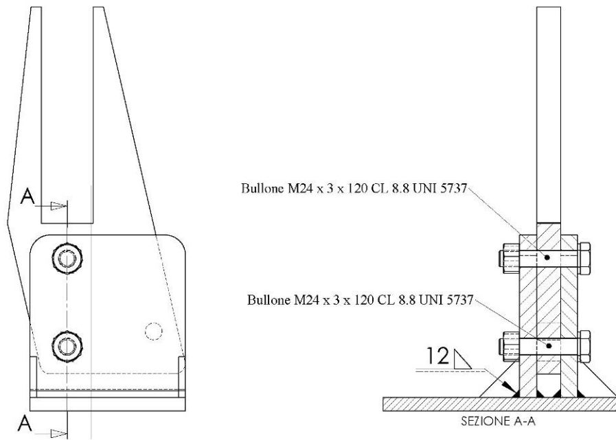
Figura 5. Assieme dell'elemento di collegamento per telaio abbattibile
