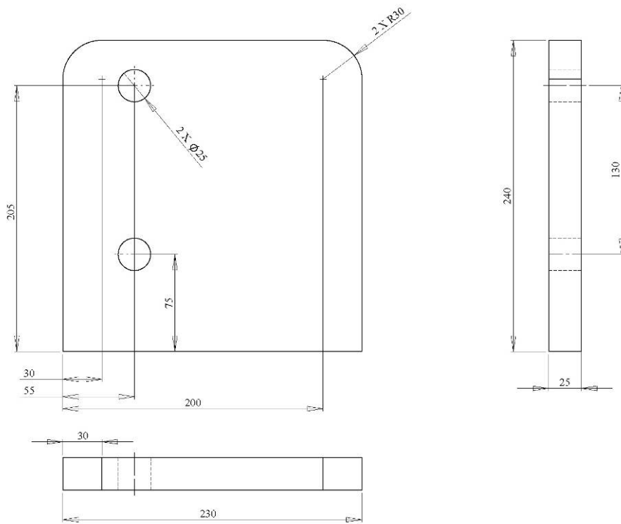
Figura 4. Piastra laterale interna per telaio abbattibile
