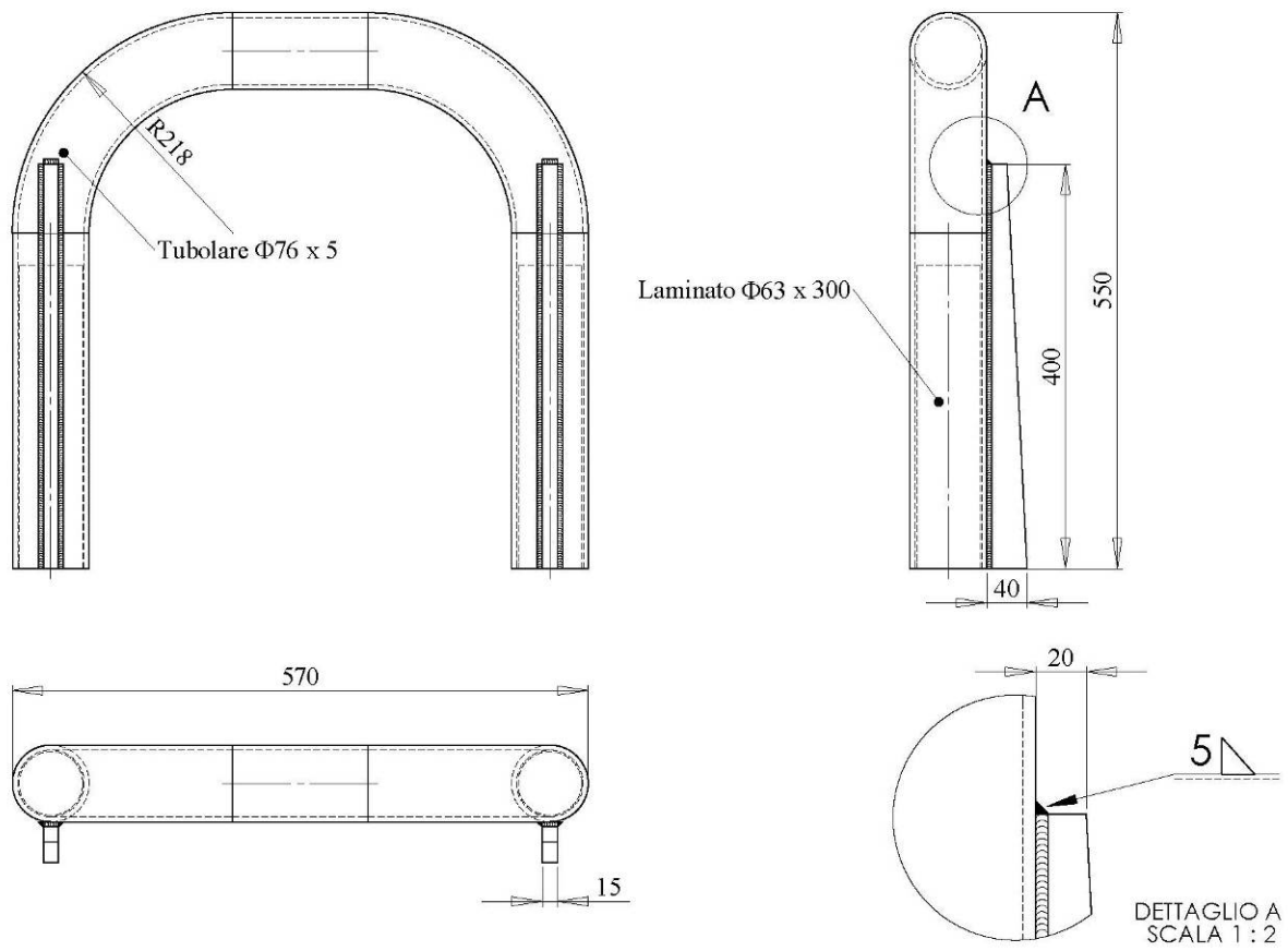
Figura 1. Telaio rigido posteriore
