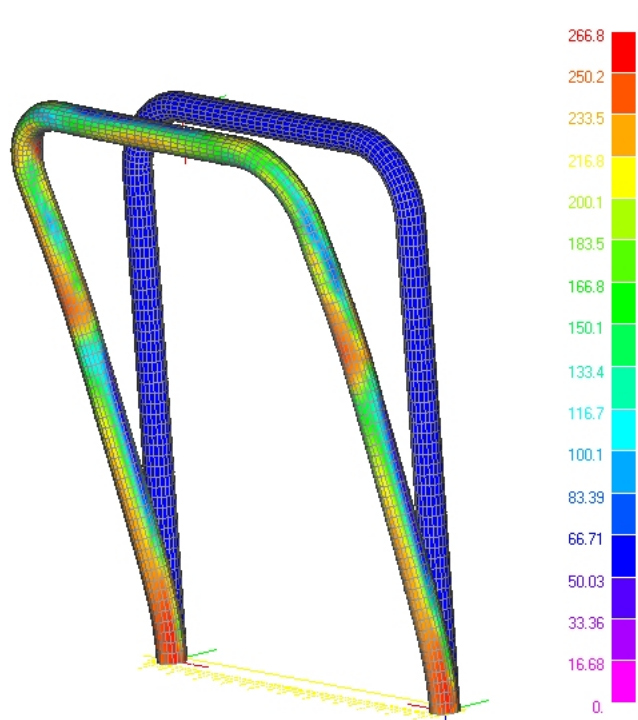
Figura 12. Carico posteriore: diagramma a falsi colori della tensione [MPa]
