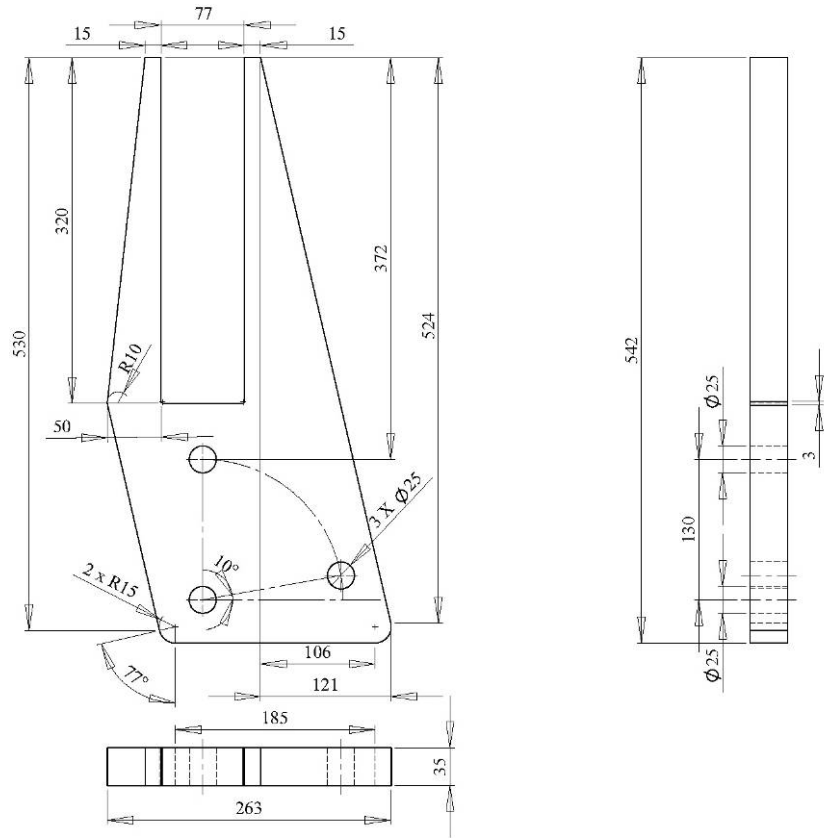
Figura 3. Piastra interna di collegamento per telaio abbattibile
