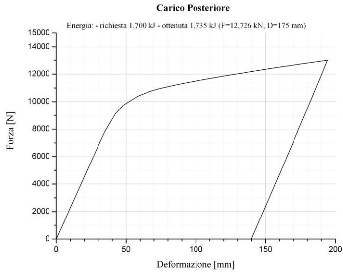
Figura 6. Carico posteriore: diagramma Forza vs. Deformazione
