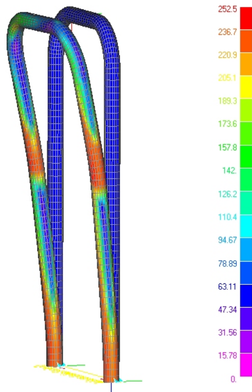
Figura 5. Carico posteriore: diagramma a falsi colori della tensione [MPa]
