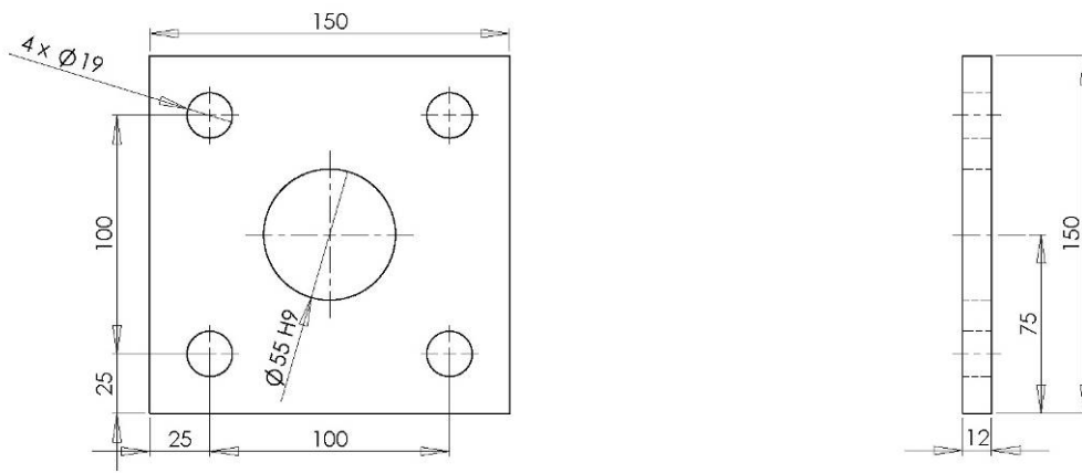
Figura 2. Piastra alla base del telaio
