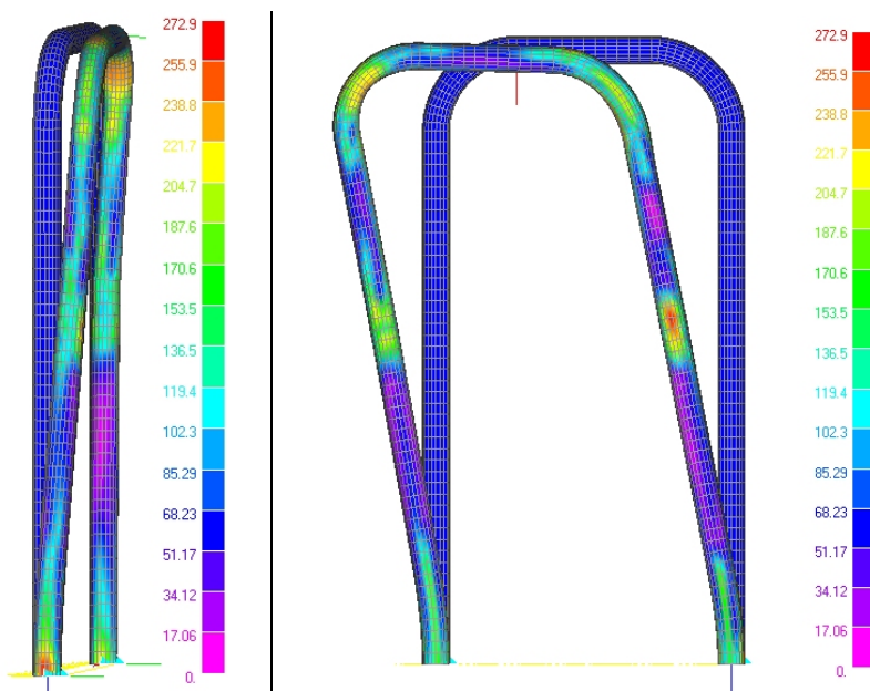
Figura 11. Deformazione residua: diagramma a falsi colori della tensione [MPa]
