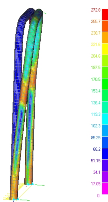
Figura 7. Carico frontale: diagramma a falsi colori della tensione [MPa]
