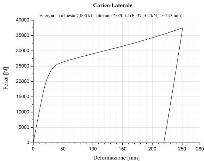
Figura 10. Carico laterale: diagramma Forza vs. Deformazione
