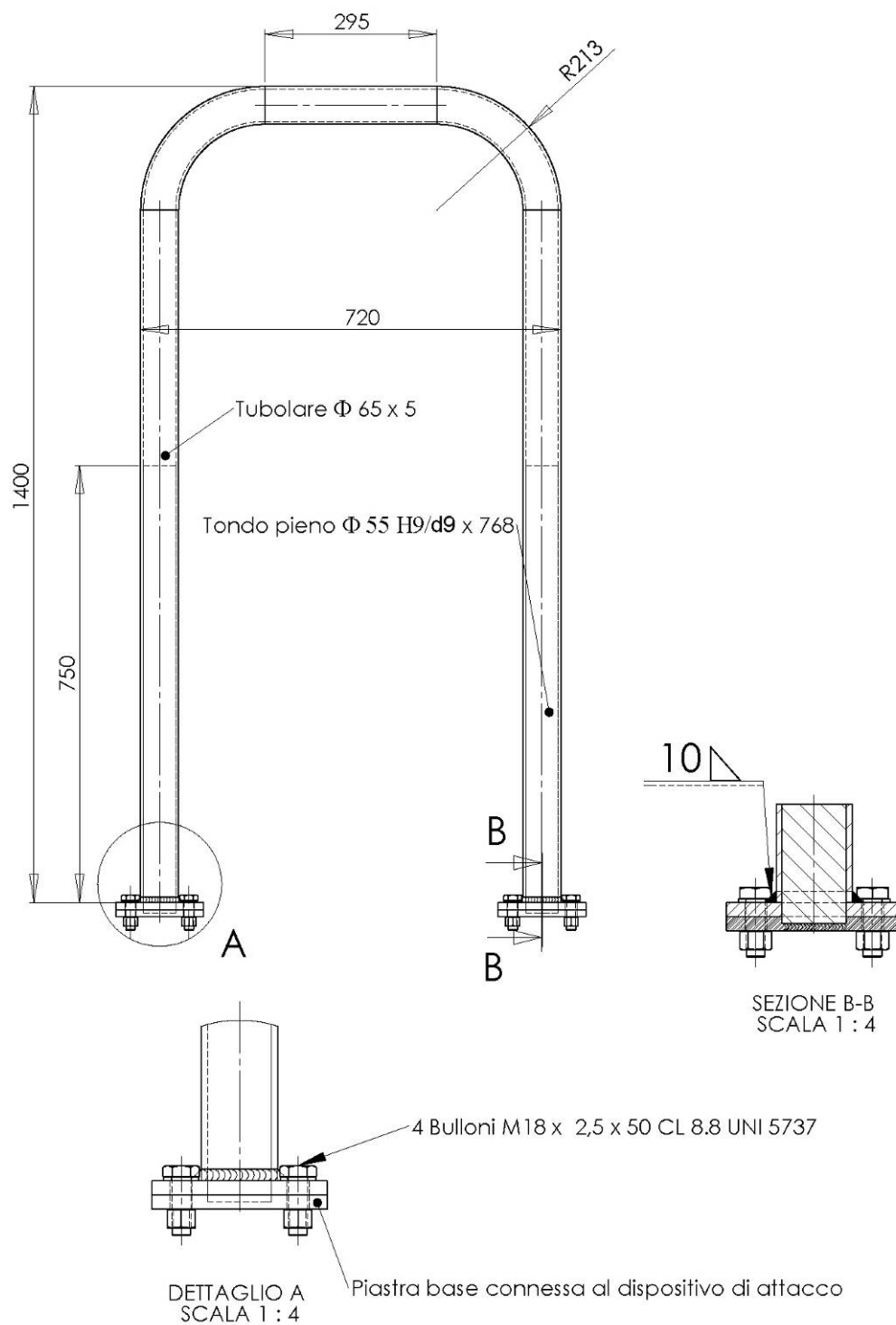
Figura 1. Telaio di protezione posteriore fisso
