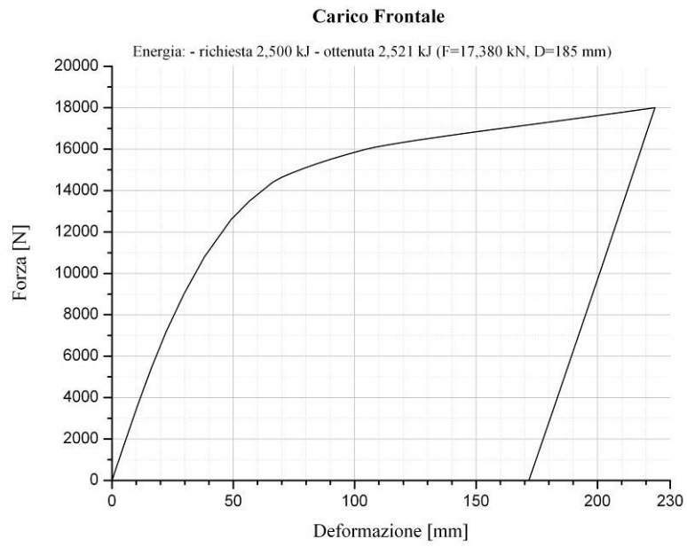
Figura 8. Carico frontale: diagramma Forza vs. Deformazione
