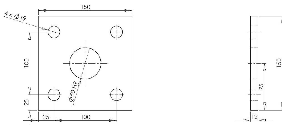
Figura 2. Piastra alla base del telaio
