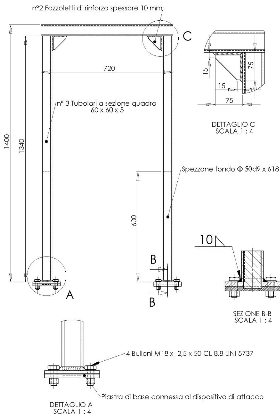
Figura 1. Telaio di protezione posteriore fisso
