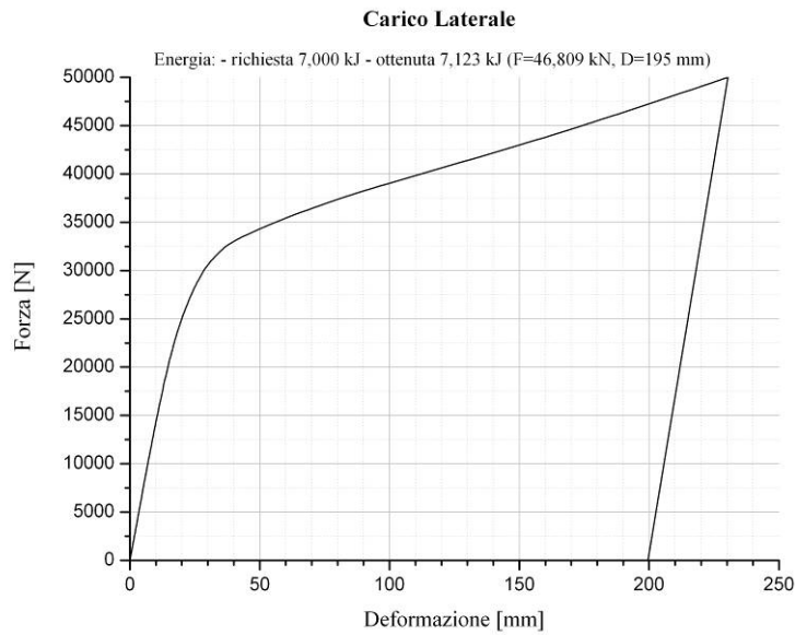
Figura 10. Carico laterale: diagramma Forza vs. Deformazione
