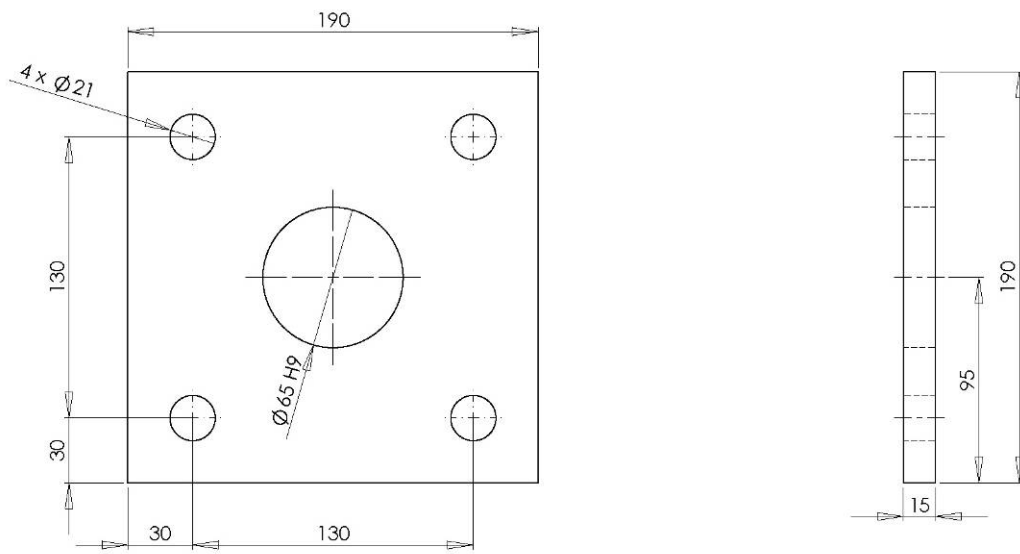
Figura 2. Piastra alla base del telaio
