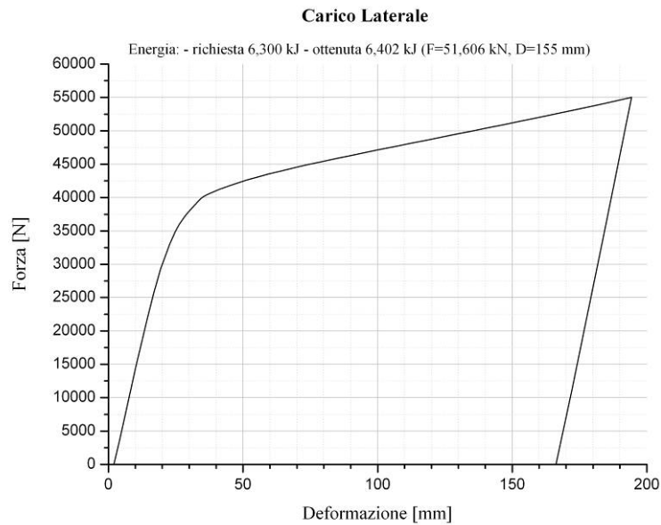
Figura 8. Carico laterale: diagramma Forza vs. Deformazione
