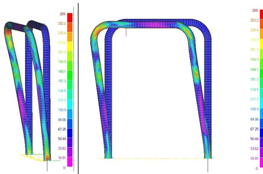
Figura 9. Deformazione residua: diagramma a falsi colori della tensione [MPa]
