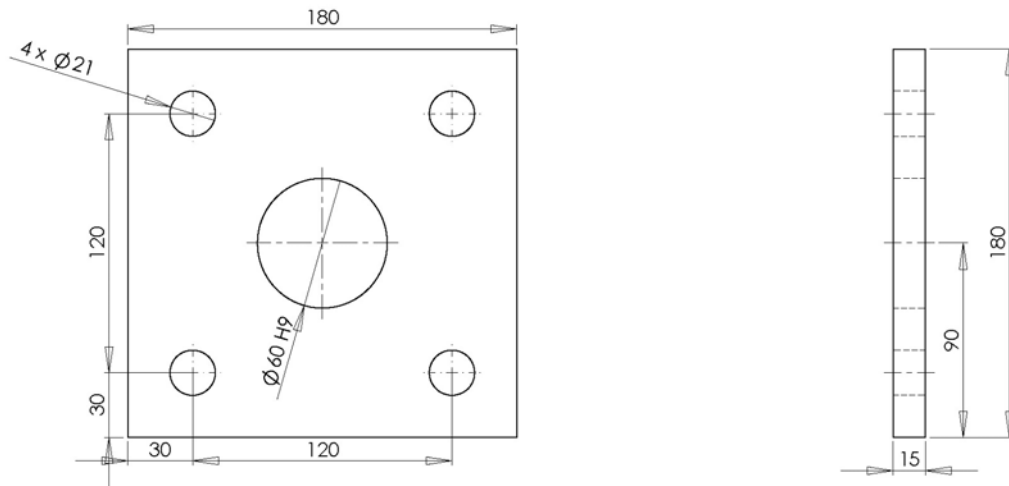
Figura 2. Piastra alla base del telaio
