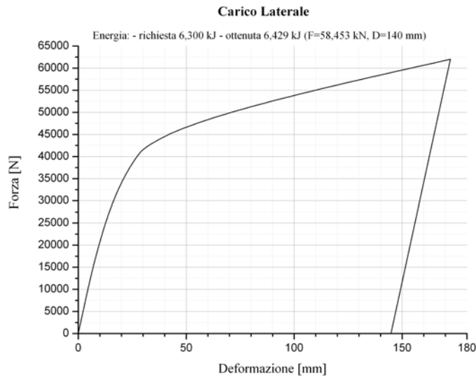
Figura 8. Carico laterale: diagramma Forza vs. Deformazione
