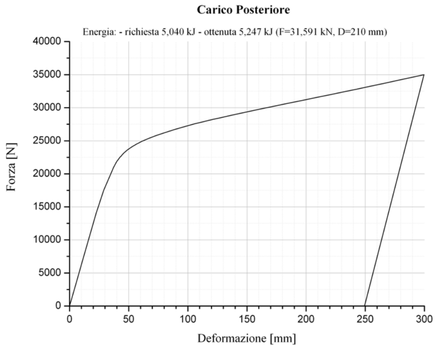
Figura 6. Carico posteriore: diagramma Forza vs. Deformazione
