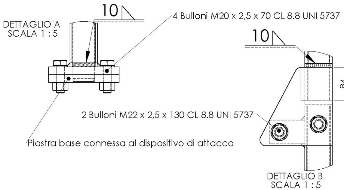
Figura 1. Telaio di protezione posteriore abbattibile
