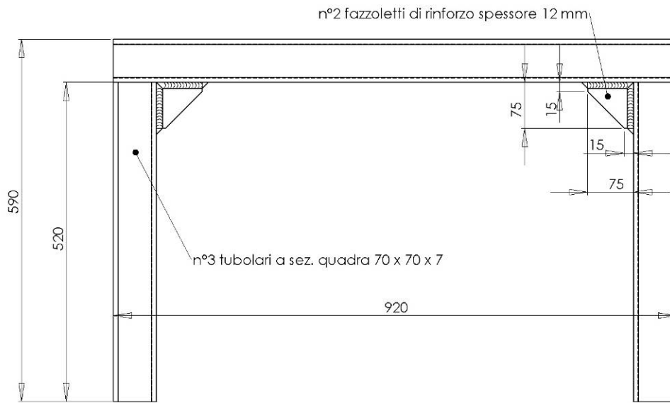
Figura 3. Dettaglio dell'arco superiore
