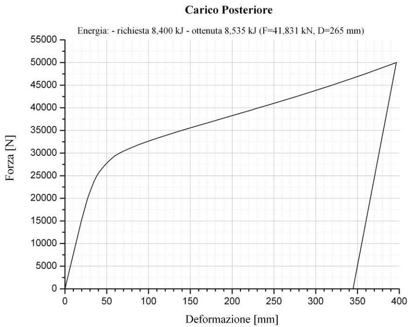
Figura 9. Carico posteriore: diagramma Forza vs. Deformazione
