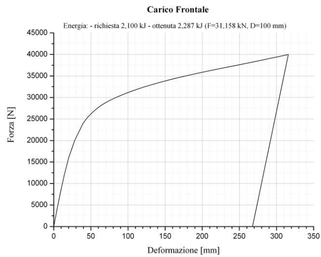
Figura 13. Carico frontale: diagramma Forza vs. Deformazione
