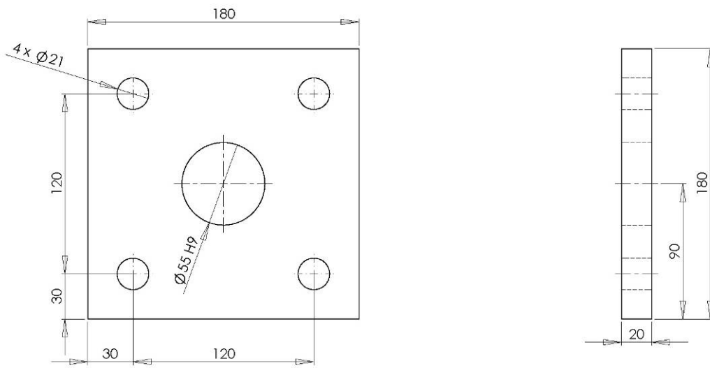
Figura 5. Piastra di base
