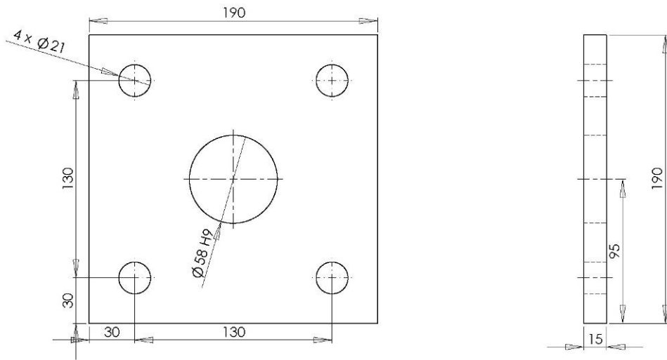
Figura 3. Piastra alla base del telaio
