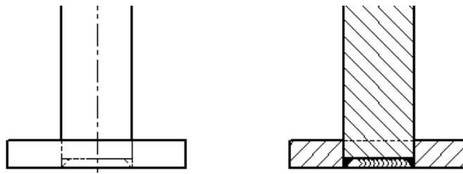
Figura 4. Saldatura spezzone tondo
