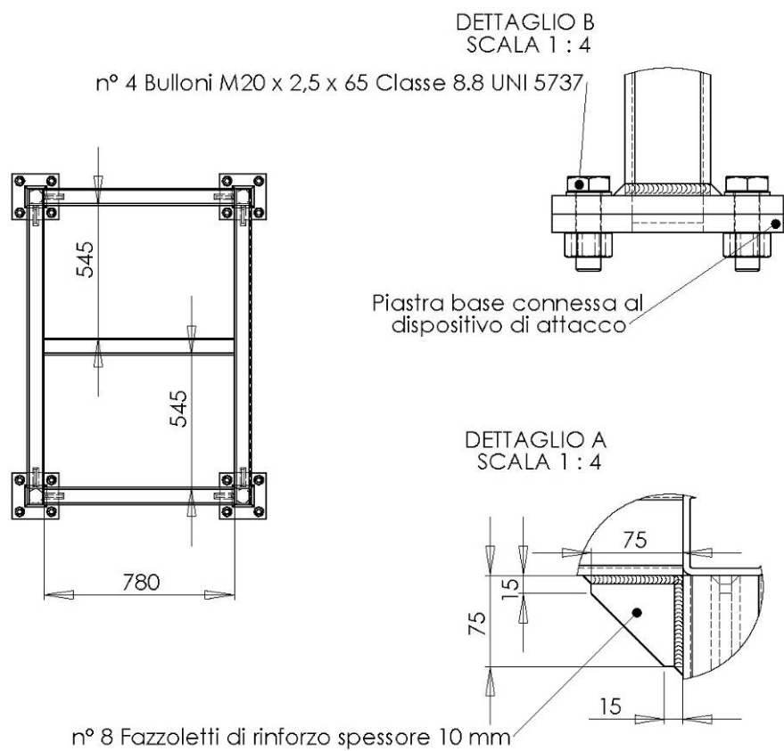
Figura 2. Telaio di protezione a quattro montanti
