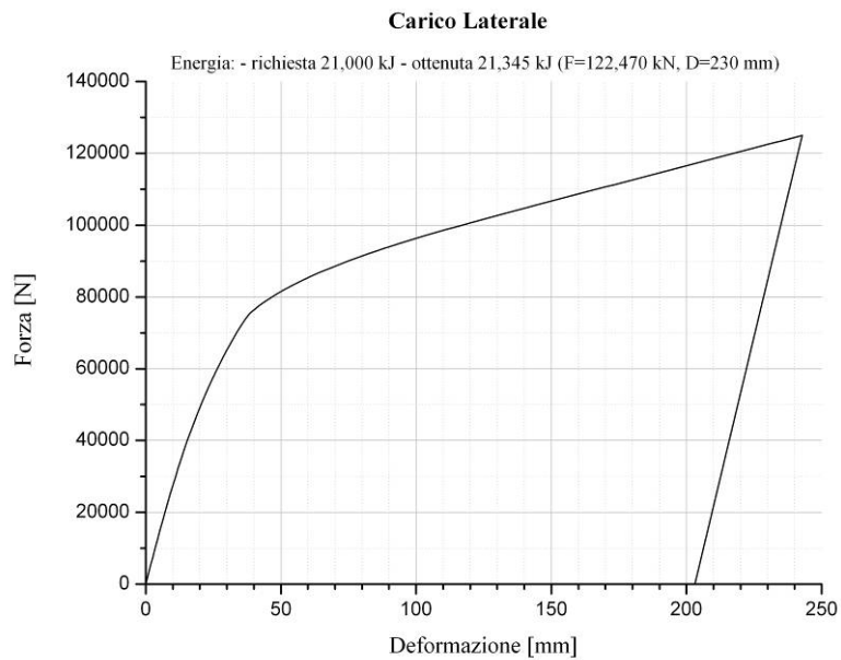
Figura 9. Carico laterale: diagramma Forza vs. Deformazione
