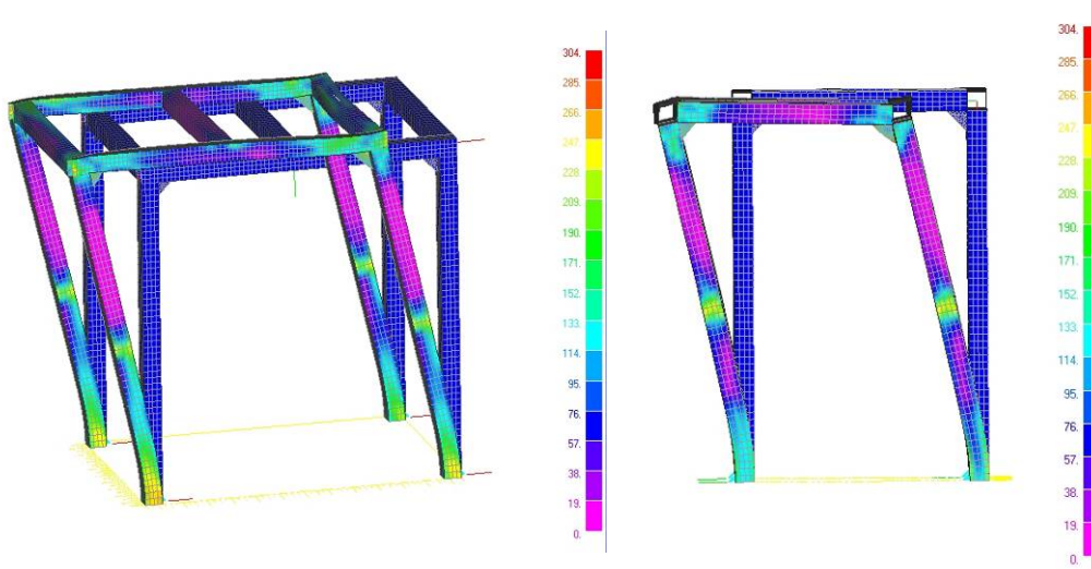
Figura 10. Deformazione residua: diagramma a falsi colori della tensione [MPa]
