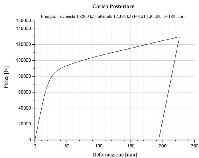
Figura 7. Carico posteriore: diagramma Forza vs. Deformazione
