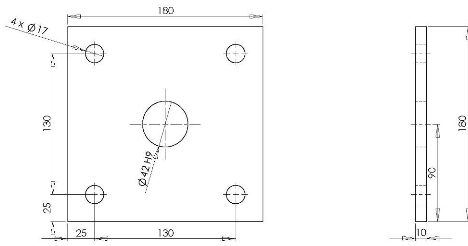
Figura 6. Piastra alla base del telaio
