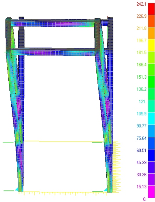
Figura 11. Carico verticale: diagramma a falsi colori della tensione [MPa]
