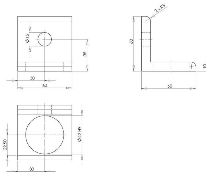
Figura 5. Piastra angolare
