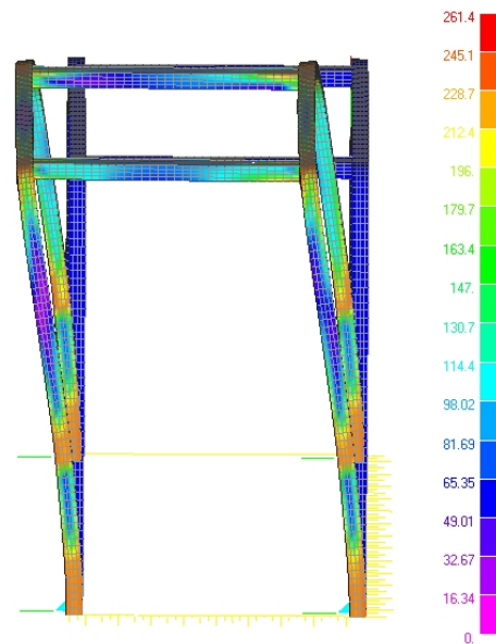
Figura 9. Carico laterale: diagramma a falsi colori della tensione [MPa]
