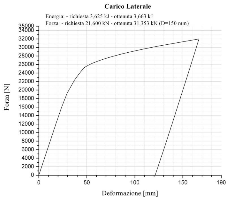
Figura 10. Carico laterale: diagramma Forza vs. Deformazione
