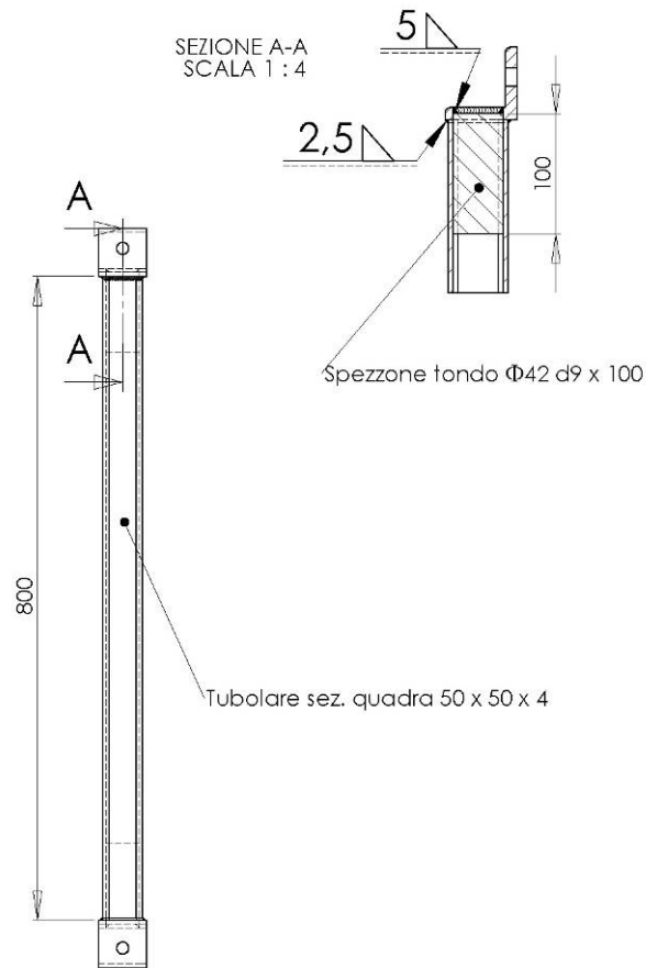
Figura 4. Traversa trasversale
