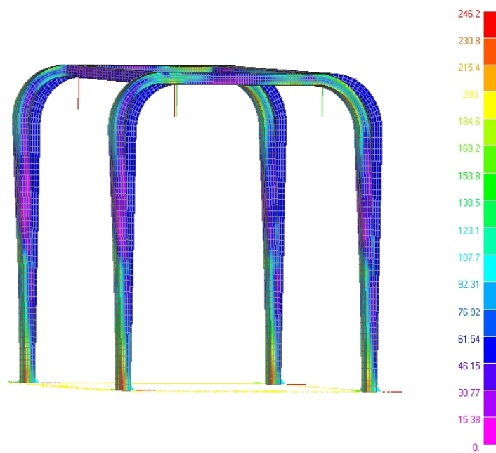
Figura 12. Carico posteriore: diagramma a falsi colori della tensione [MPa]
