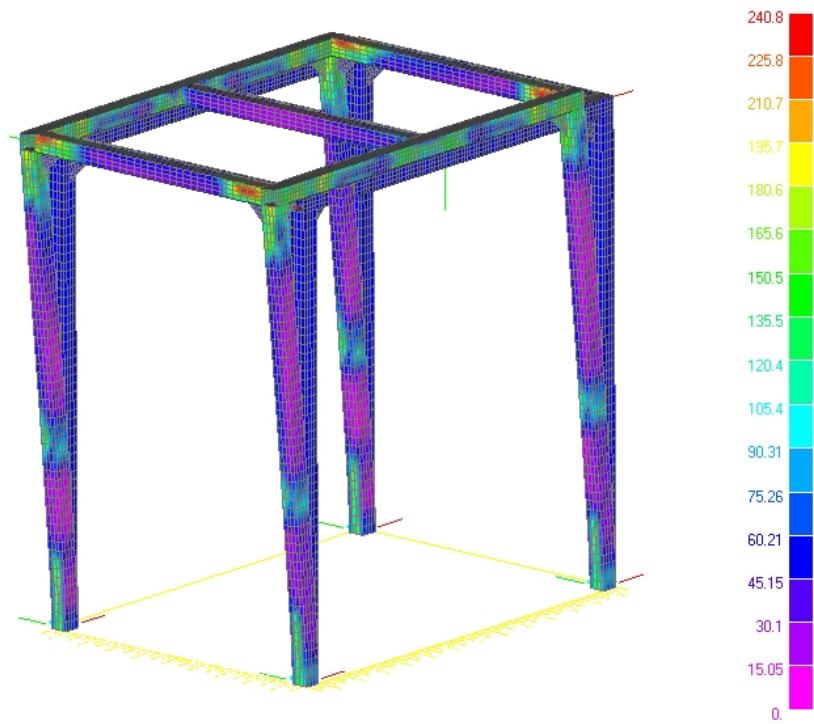
Figura 8. Carico verticale: diagramma a falsi colori della tensione [MPa]
