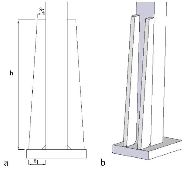
Figura 5. Disposizione flangie di rinforzo
