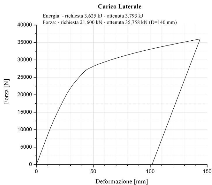
Figura 7. Carico laterale: diagramma Forza vs. Deformazione
