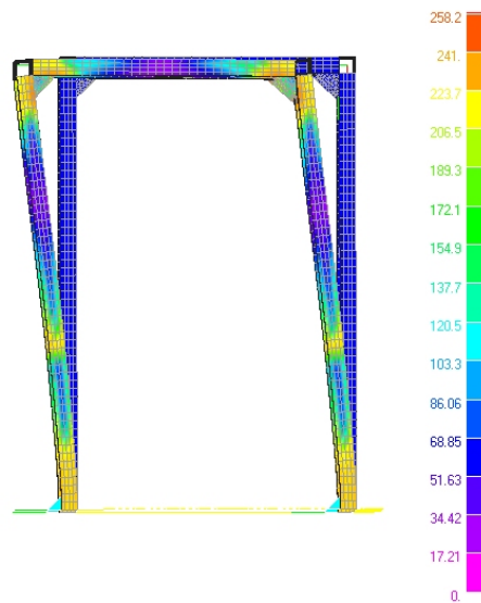
Figura 6. Carico laterale: diagramma a falsi colori della tensione [MPa]
