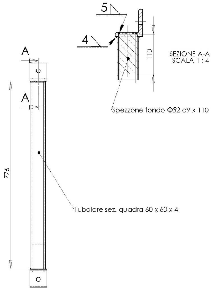
Figura 4. Traversa trasversale
