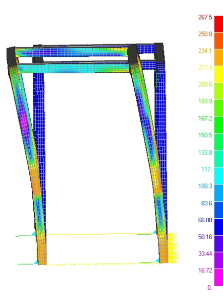
Figura 9. Carico laterale: diagramma a falsi colori della tensione [MPa]
