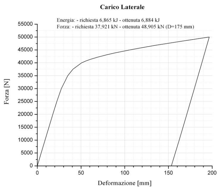
Figura 10. Carico laterale: diagramma Forza vs. Deformazione
