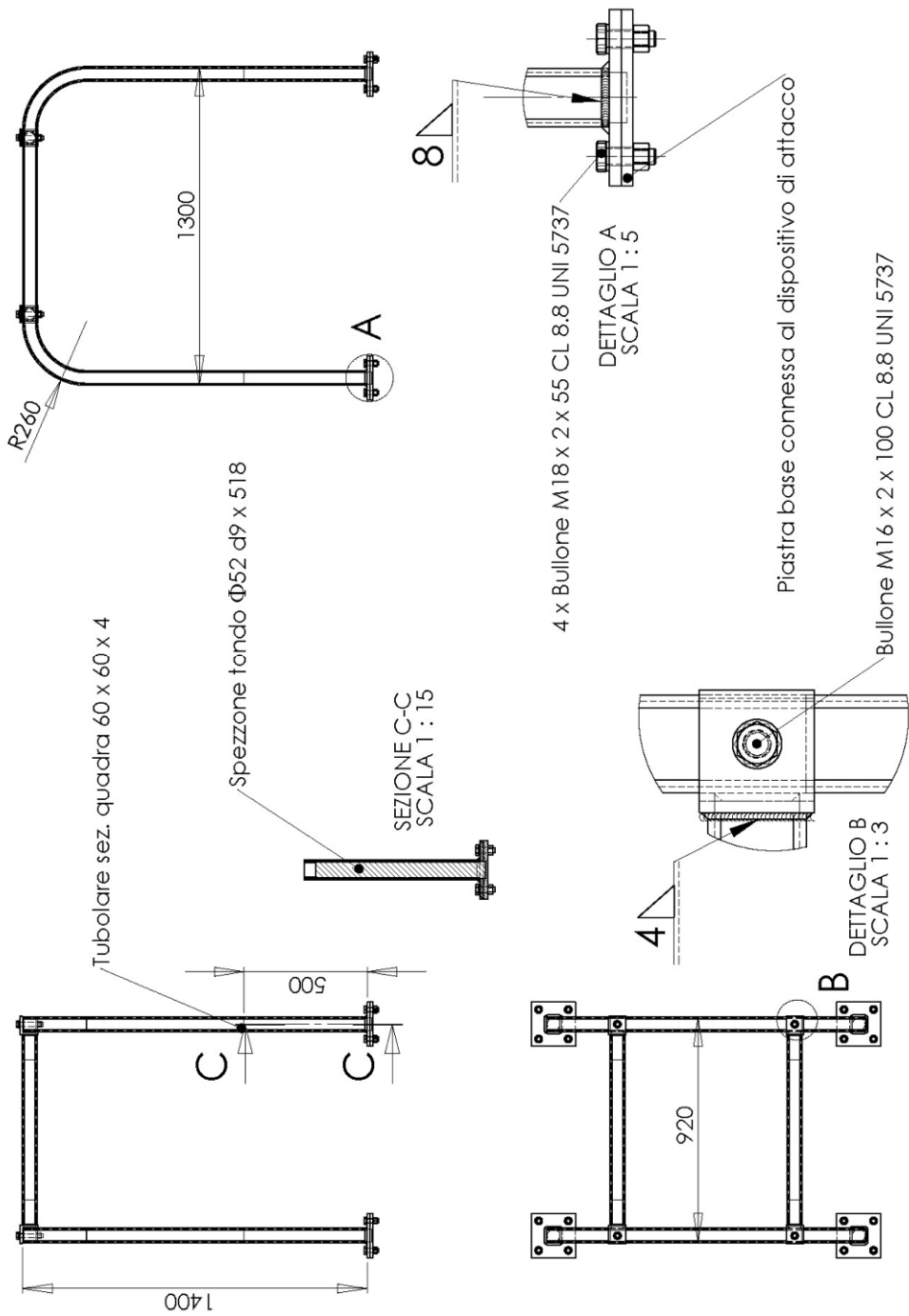
Figura 2. Telaio di protezione a quattro montanti
