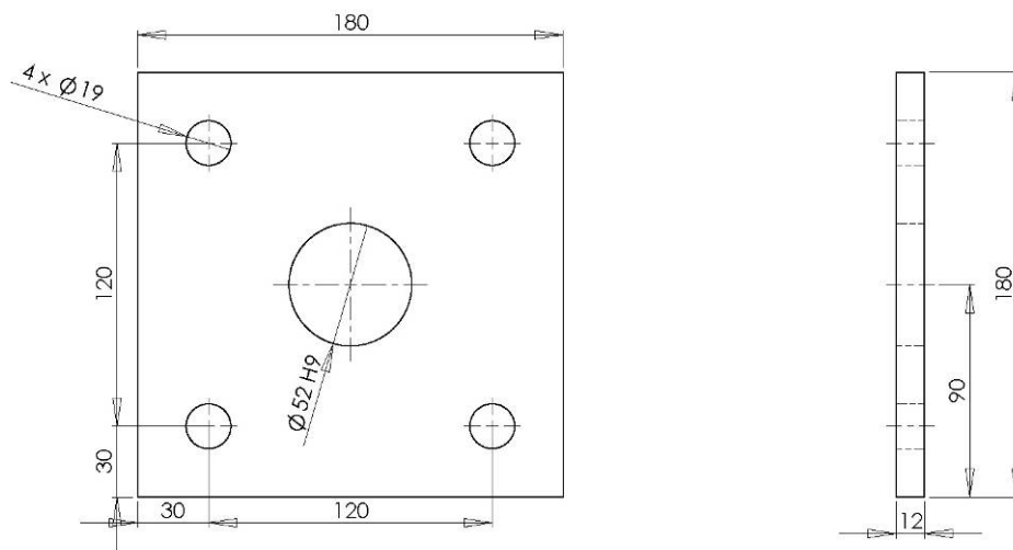
Figura 6. Piastra alla base del telaio
