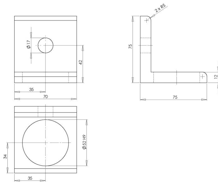
Figura 5. Piastra angolare
