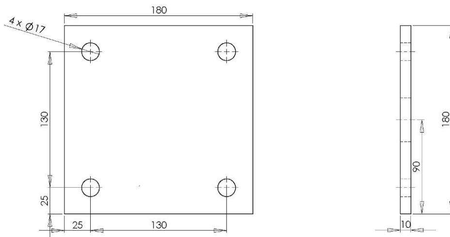
Figura 7. Piastra alla base del telaio
