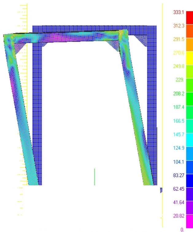
Figura 11. Carico verticale: diagramma a falsi colori della tensione [MPa]
