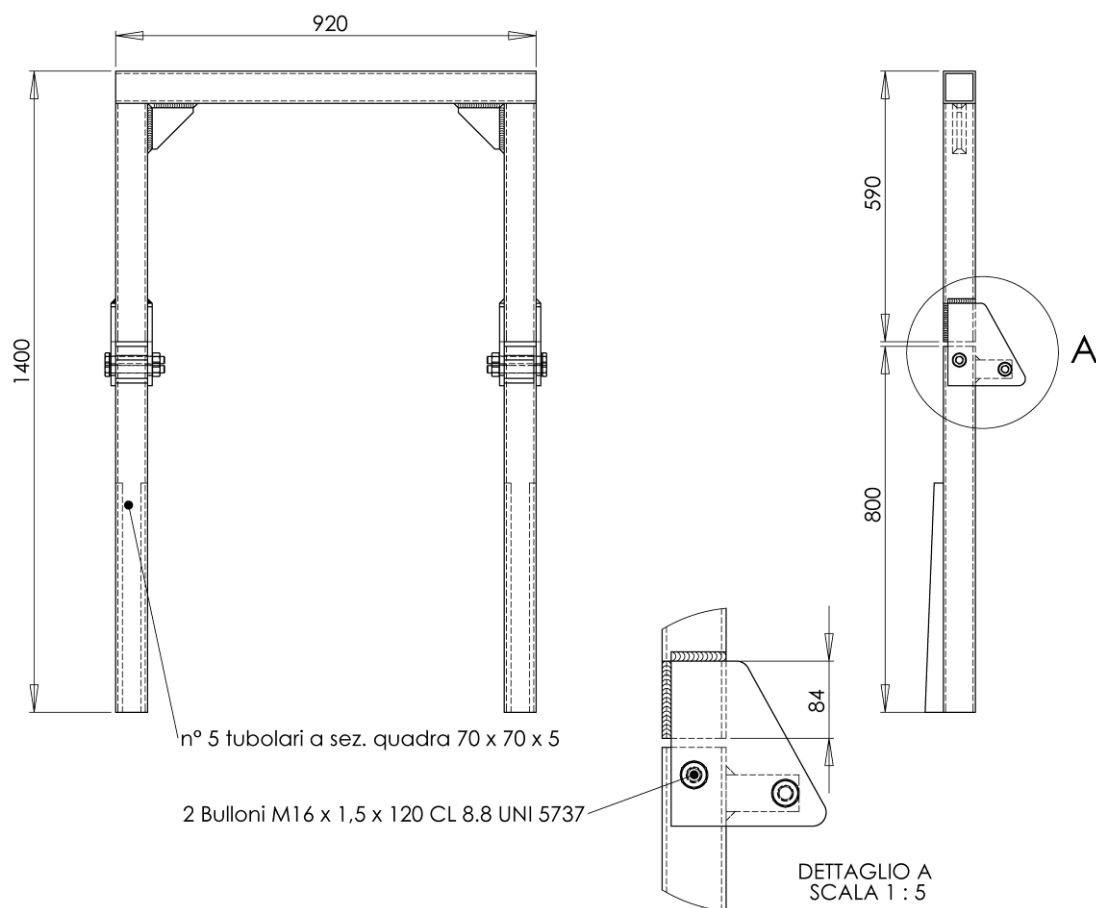
Figura 1. Telaio di protezione posteriore abbattibile
