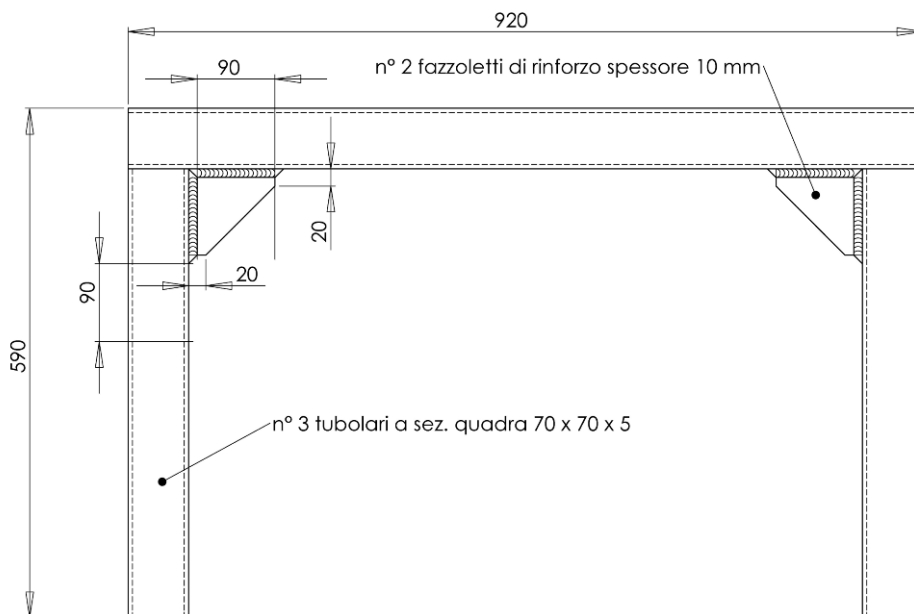
Figura 3. Arco abbattibile
