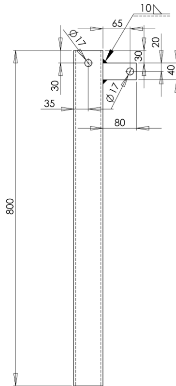
Figura 2. Montante
