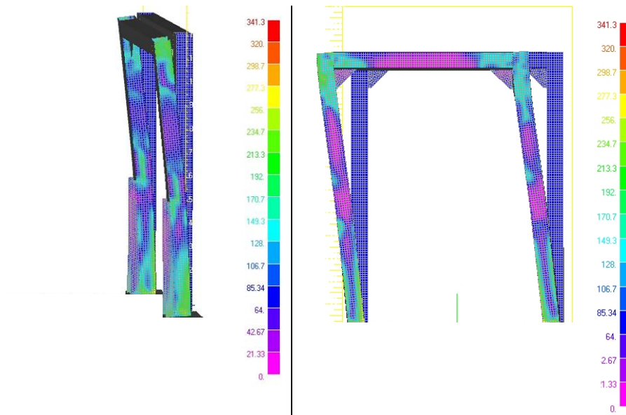
Figura 13. Deformazione residua: diagramma a falsi colori della tensione [MPa]
