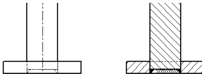
Figura 8. Saldatura spezzone tondo
