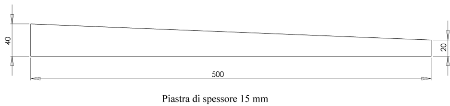
Figura 5. Flangia di rinforzo dei montanti del telaio (due per montante)
