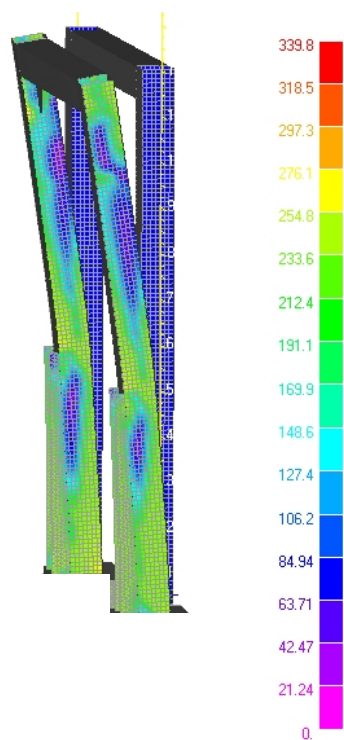
Figura 12. Carico posteriore: diagramma a falsi colori della tensione [MPa]
