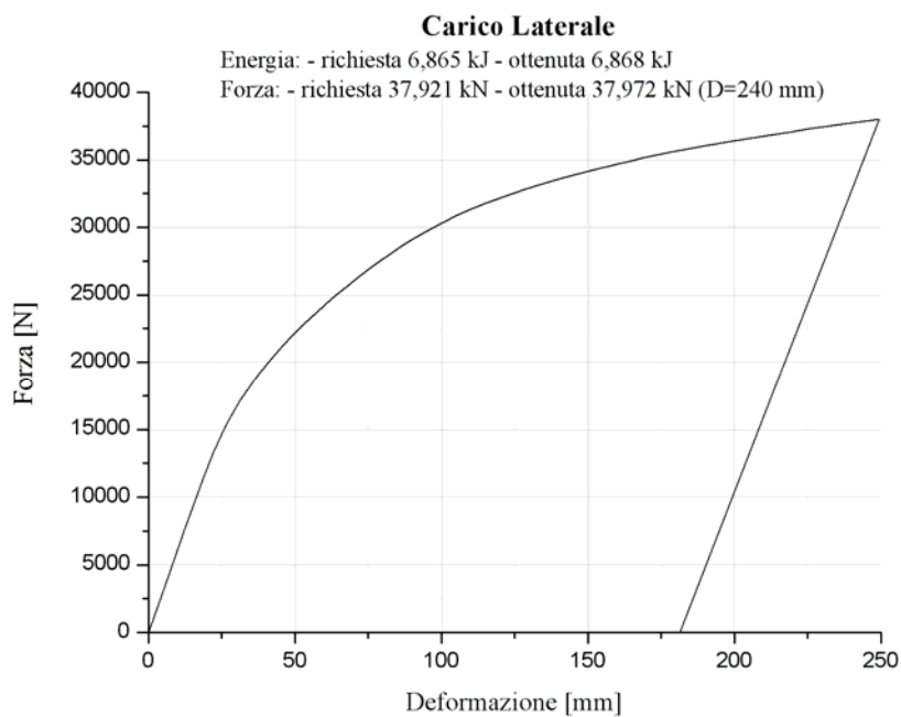
Figura 10. Carico laterale: diagramma Forza vs. Deformazione
