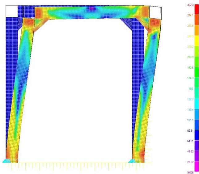
Figura 6. Carico laterale: diagramma a falsi colori della tensione [MPa]
