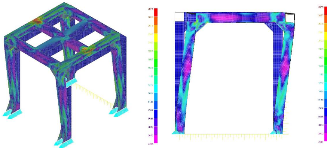
Figura 10. Deformazione residua: diagramma a falsi colori della tensione [MPa]
