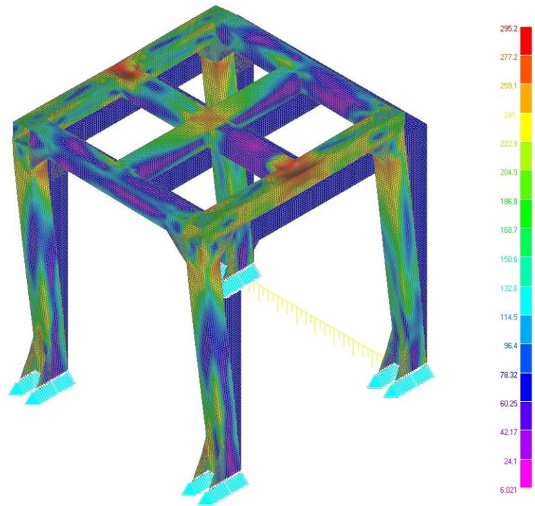
Figura 8. Carico verticale: diagramma a falsi colori della tensione [MPa]
