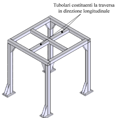
Figura 2. Vista complessiva del telaio di protezione
