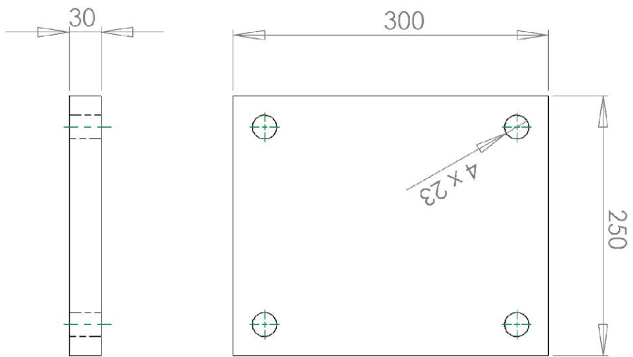
Figura 4. Piastra alla base del telaio
