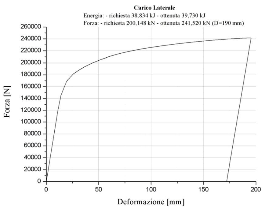
Figura 7. Carico laterale: diagramma Forza vs. Deformazione
