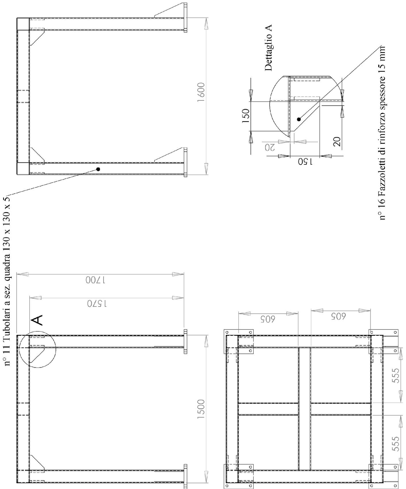
Figura 3. Telaio di protezione a quattro montanti
