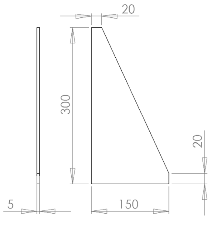
Figura 5. Flange alla base dei montanti
