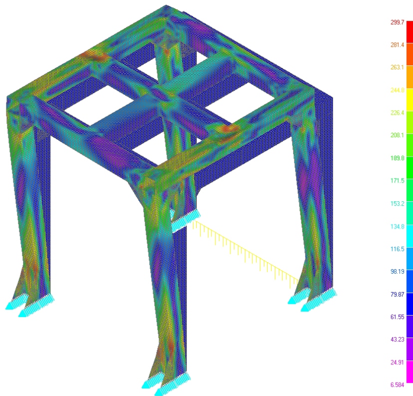
Figura 9. Carico posteriore: diagramma a falsi colori della tensione [MPa]
