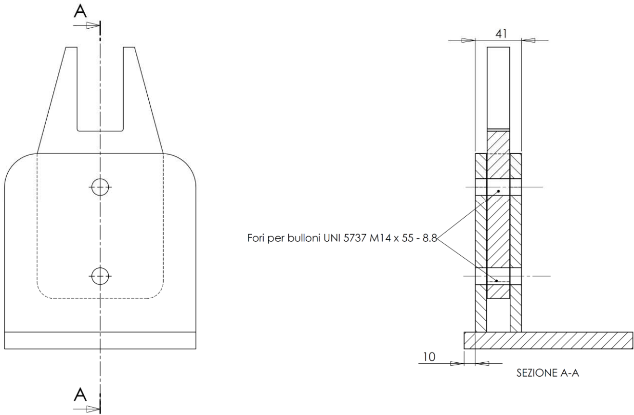
Figura 5. Assieme dell'elemento di collegamento per telaio fisso
