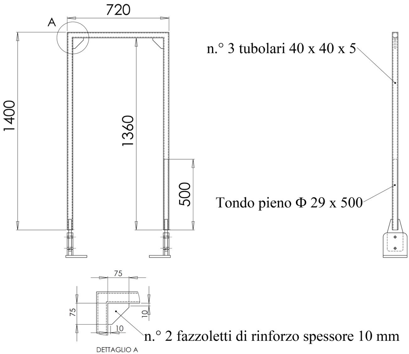
Figura 2. Telaio di protezione anteriore fisso
