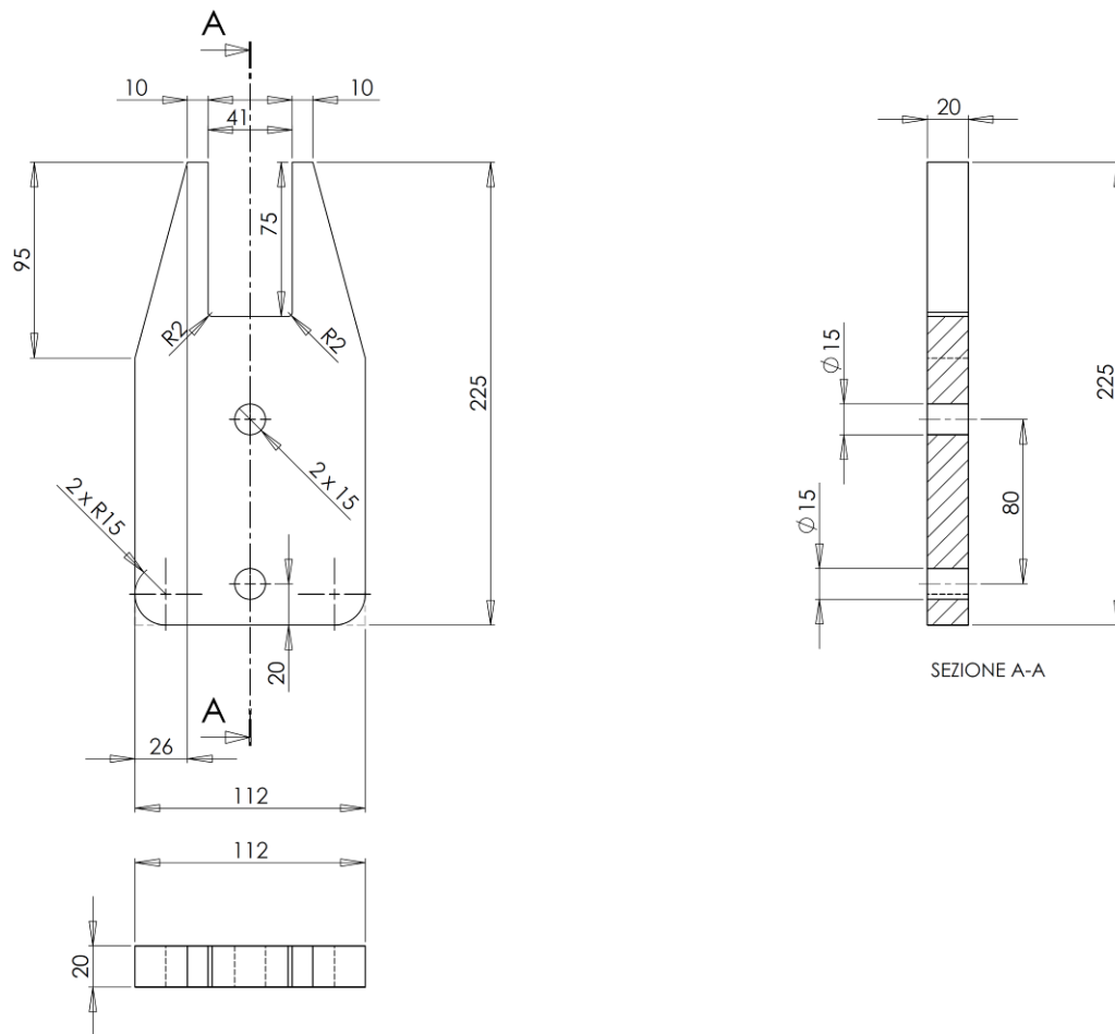
Figura 3. Piastra interna di collegamento per telaio fisso
