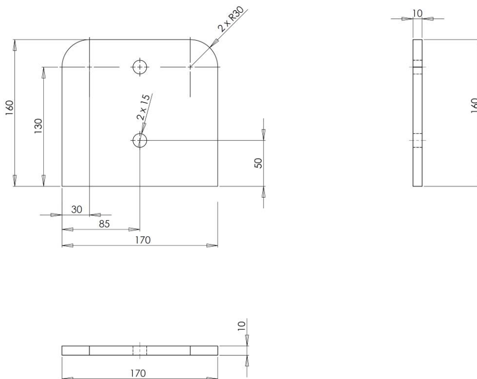
Figura 4. Piastra laterale per telaio fisso
