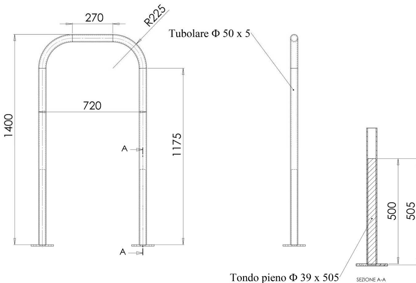
Figura 1. Telaio di protezione posteriore fisso
