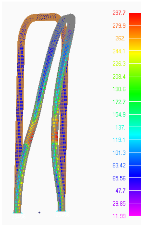
Figura 7. Carico frontale: diagramma a falsi colori della tensione [MPa]
