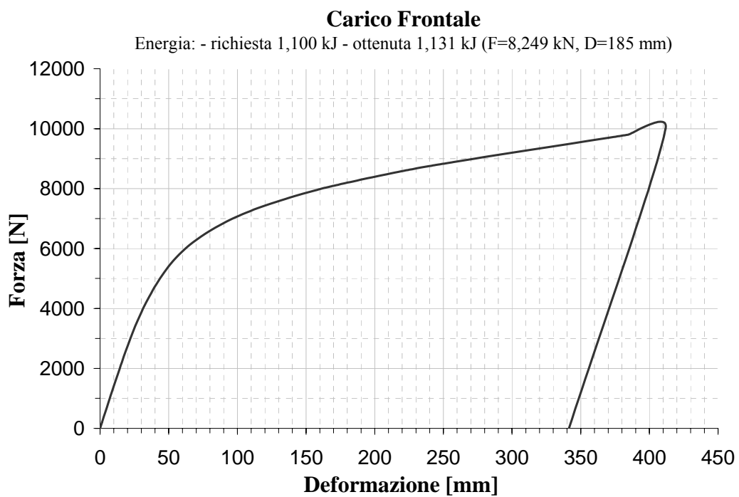
Figura 8. Carico frontale: diagramma Forza vs. Deformazione
