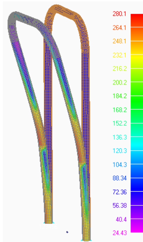
Figura 5. Carico posteriore: diagramma a falsi colori della tensione [MPa]
