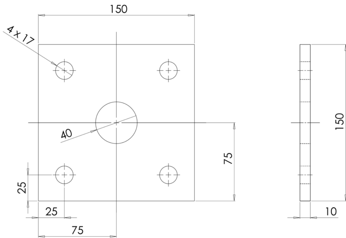
Figura 2. Piastra alla base del telaio
