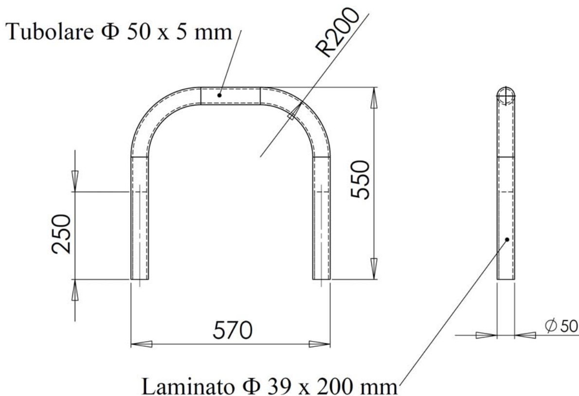
Figura 1. Telaio rigido posteriore
