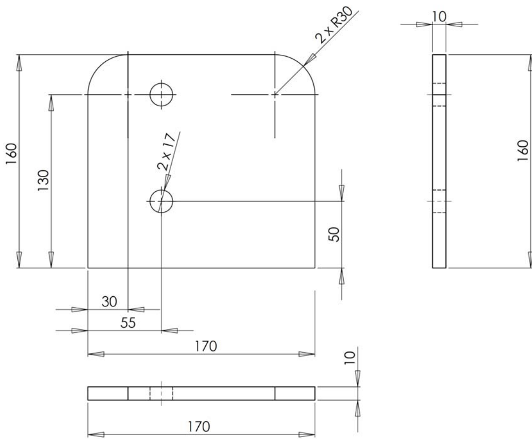
Figura 4. Piastra laterale interna per telaio abbattibile
