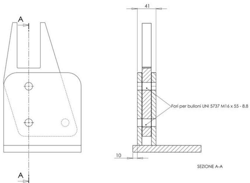
Figura 5. Assieme dell'elemento di collegamento per telaio abbattibile
