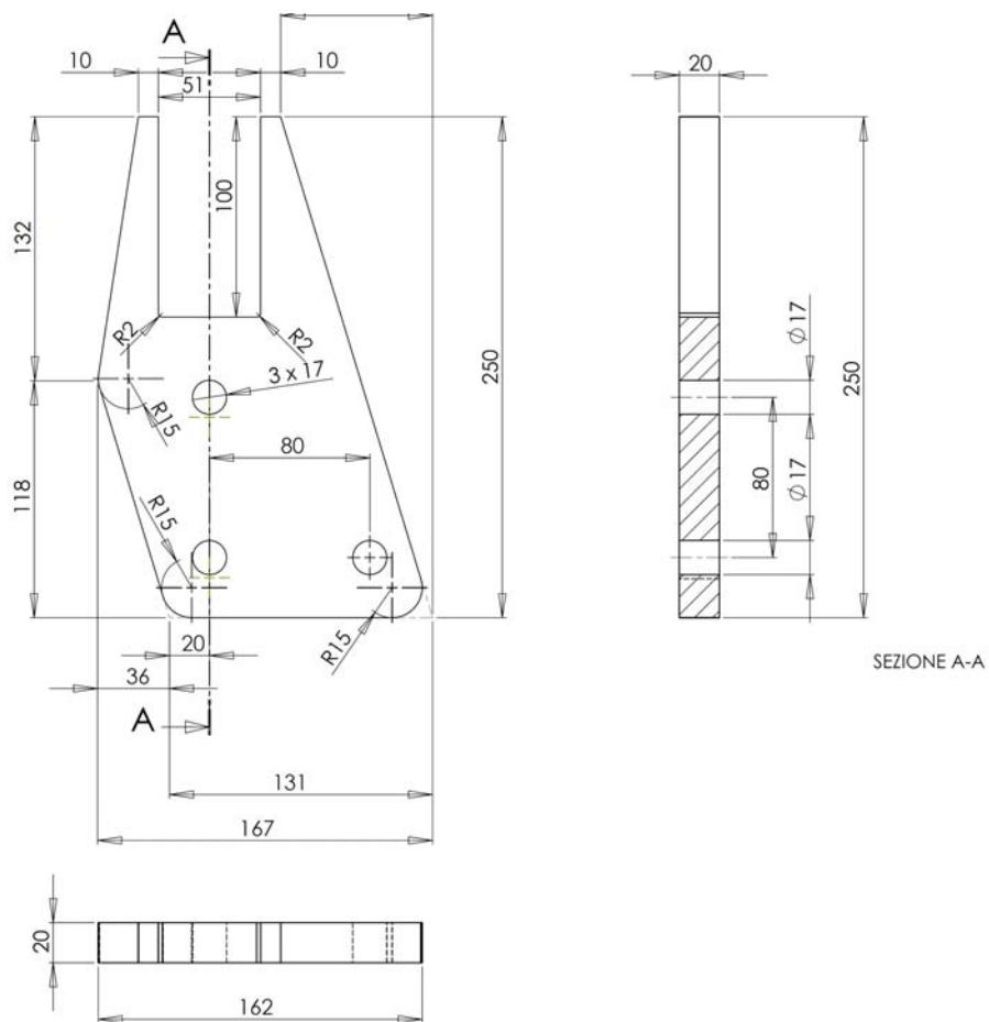
Figura 3. Piastra interna di collegamento per telaio abbattibile
