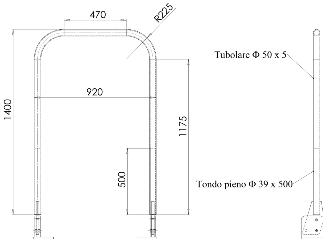
Figura 2. Telaio di protezione anteriore abbattibile
