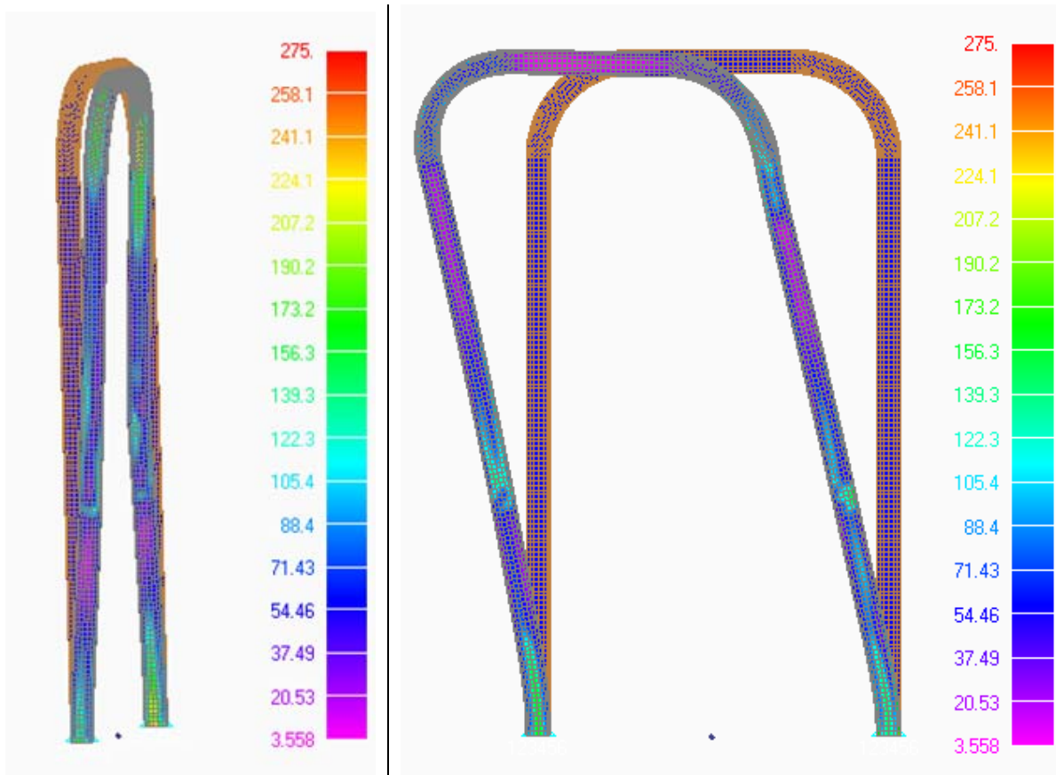
Figura 8. Deformazione residua: diagramma a falsi colori della tensione [MPa]
