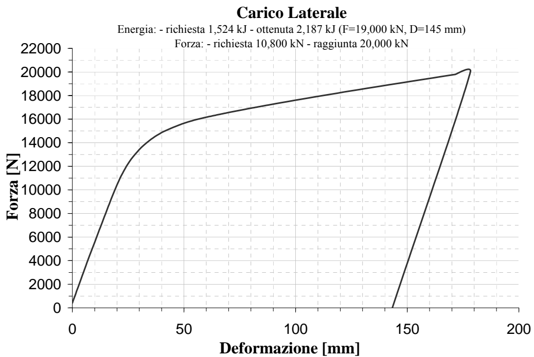
Figura 6. Carico laterale: diagramma Forza vs. Deformazione
