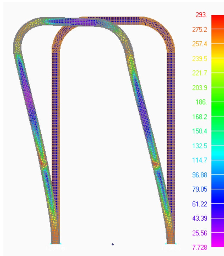
Figura 5. Carico laterale: diagramma a falsi colori della tensione [MPa]
