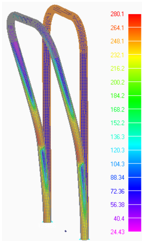
Figura 7. Carico posteriore: diagramma a falsi colori della tensione [MPa]
