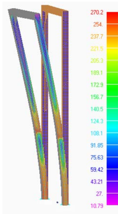
Figura 7. Carico posteriore: diagramma a falsi colori della tensione [MPa]
