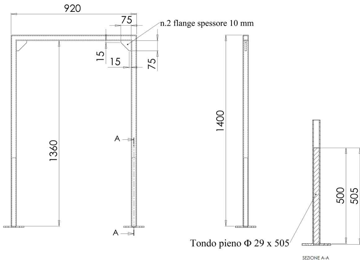
Figura 1. Telaio di protezione
