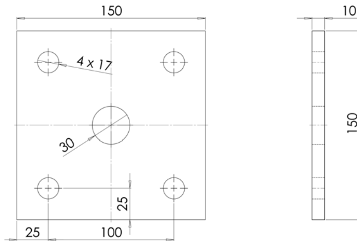
Figura 2. Piastra alla base del telaio
