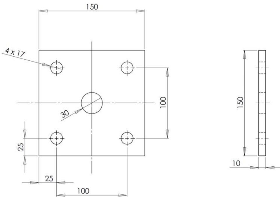
Figura 5. Piastra alla base del telaio
