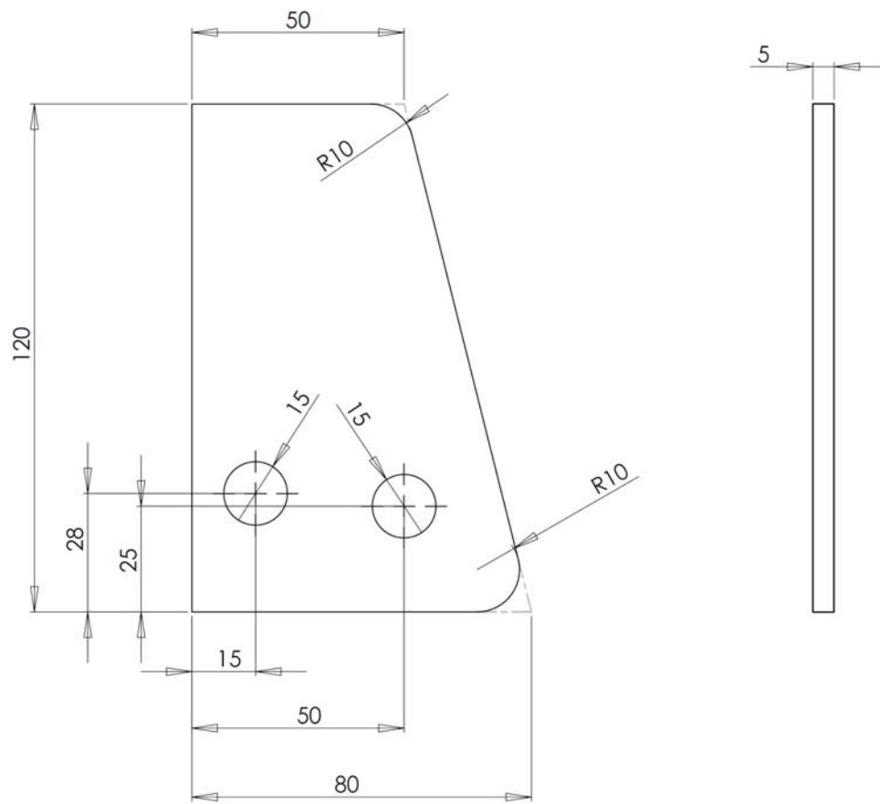
Figura 4. Piastra laterale
