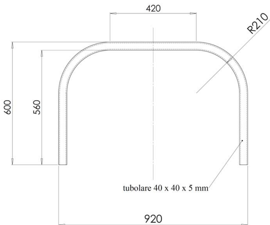
Figura 3. Arco abbattibile
