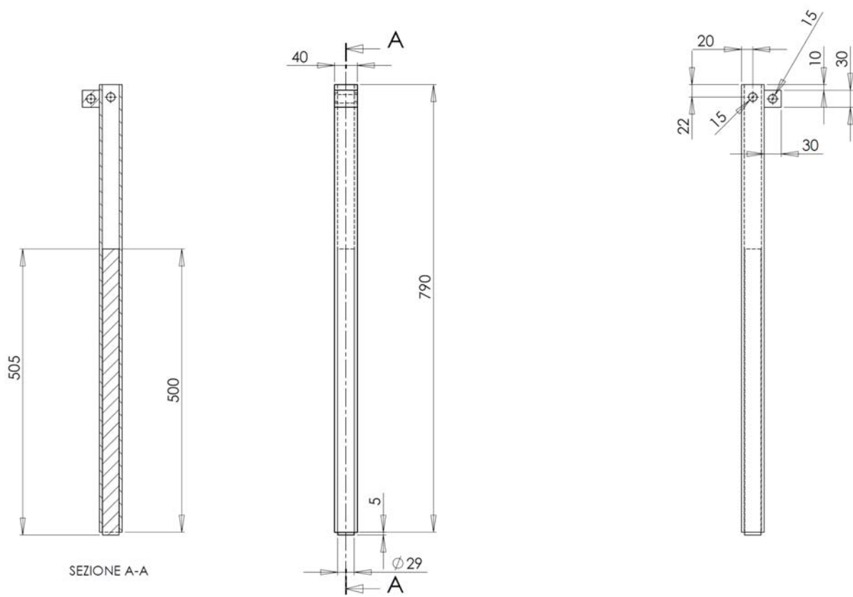
Figura 2. Montante
