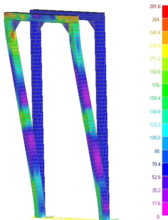
Figura 7. Carico verticale: diagramma a falsi colori della tensione [MPa]
