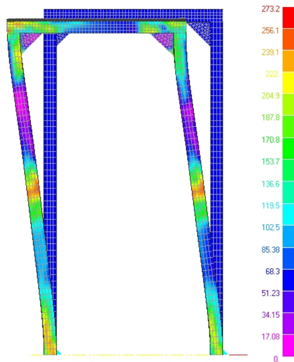
Figura 5. Carico laterale: diagramma a falsi colori della tensione [MPa]
