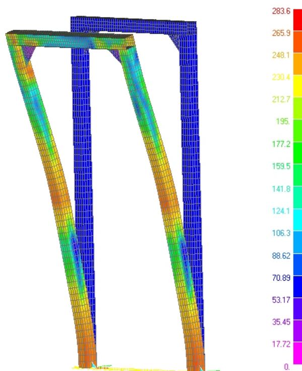
Figura 8. Carico posteriore: diagramma a falsi colori della tensione [MPa]
