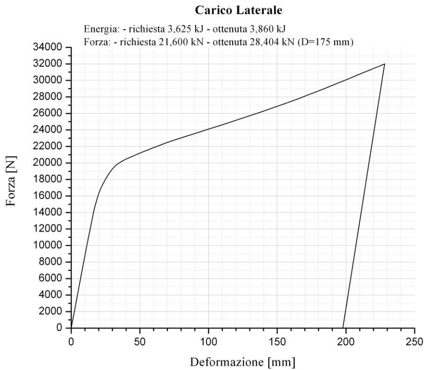
Figura 6. Carico laterale: diagramma Forza vs. Deformazione
