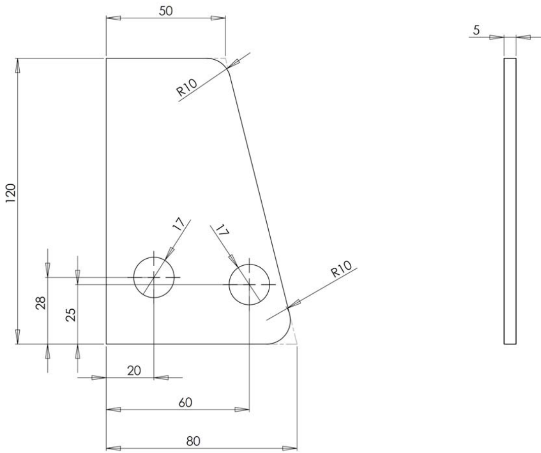
Figura 4. Piastra laterale
