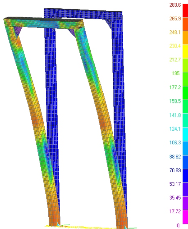
Figura 11. Carico posteriore: diagramma a falsi colori della tensione [MPa]
