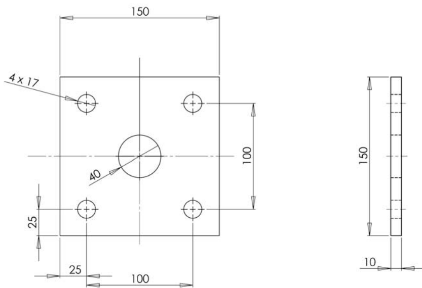
Figura 5. Piastra alla base del telaio
