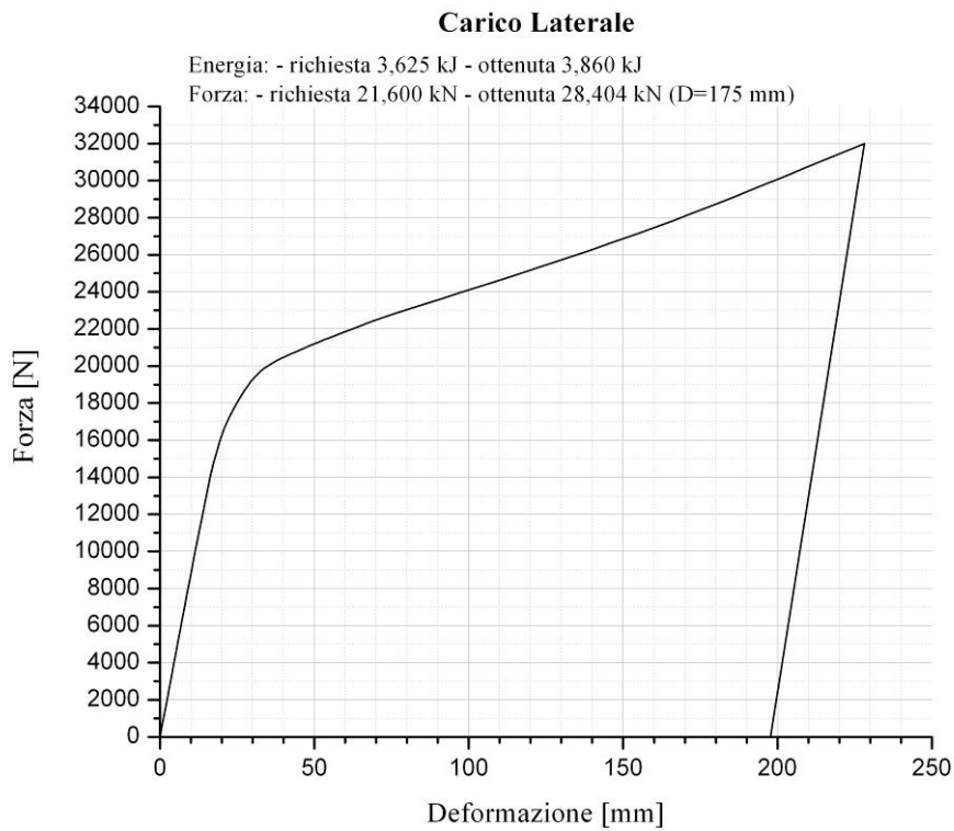
Figura 9. Carico laterale: diagramma Forza vs. Deformazione
