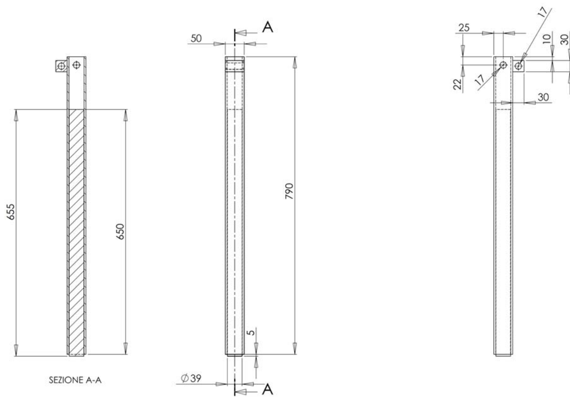
Figura 2. Montante
