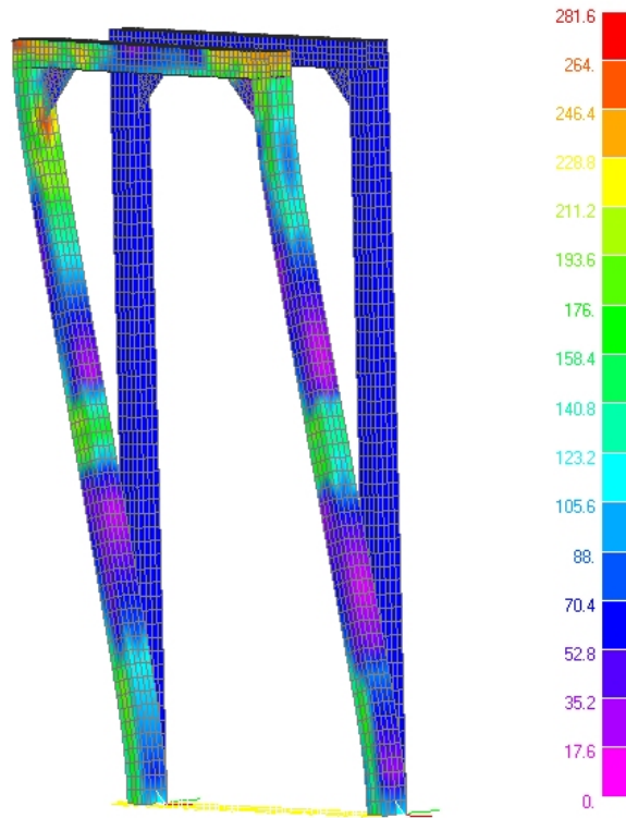
Figura 10. Carico verticale: diagramma a falsi colori della tensione [MPa]
