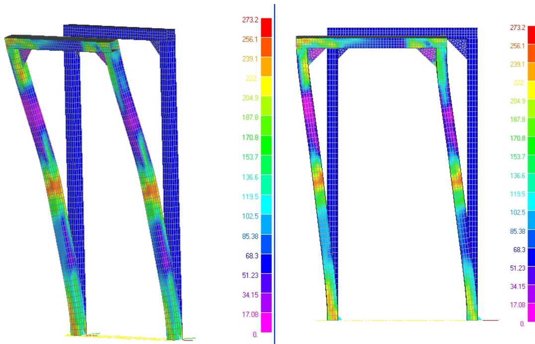
Figura 12. Deformazione residua: diagramma a falsi colori della tensione [MPa]
