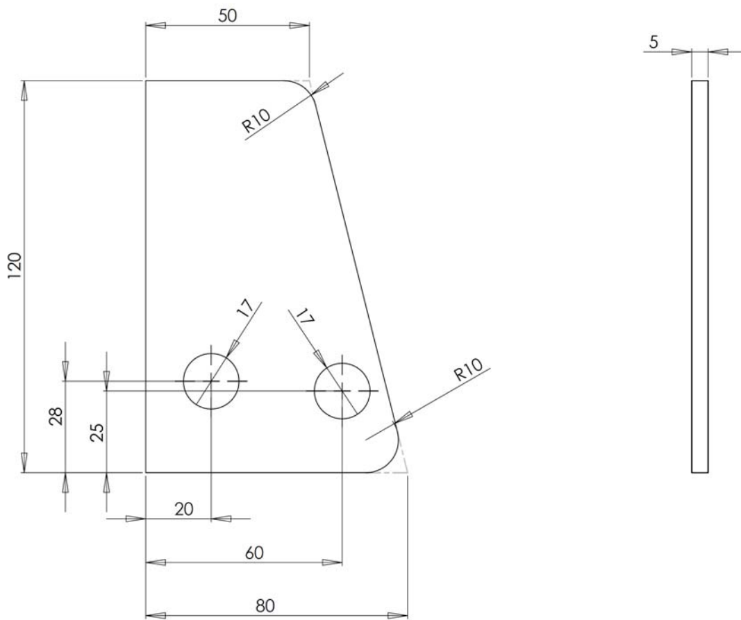
Figura 4. Piastra laterale
