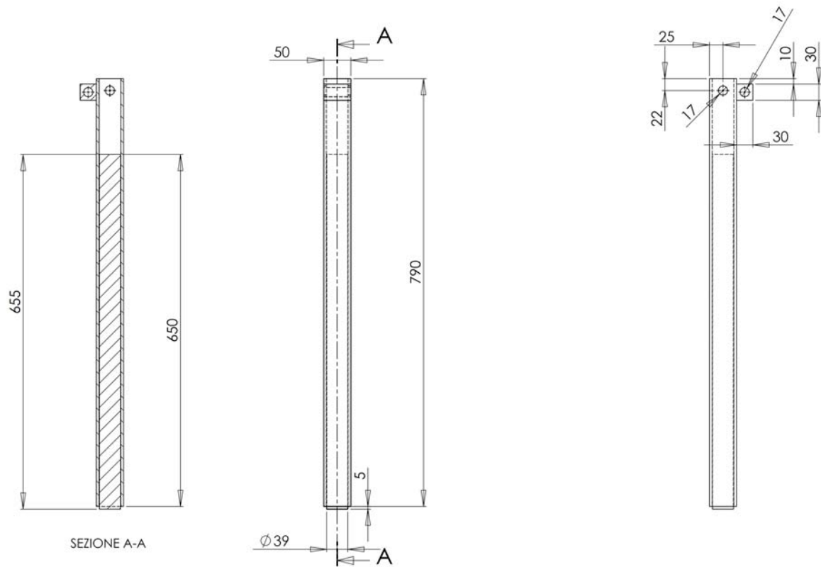
Figura 2. Montante
