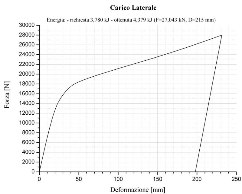
Figura 14. Carico laterale: diagramma Forza vs. Deformazione
