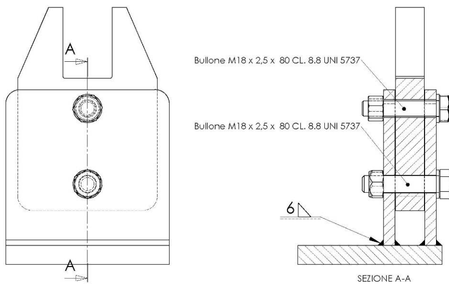
Figura 5. Assieme dell'elemento di collegamento per telaio fisso
