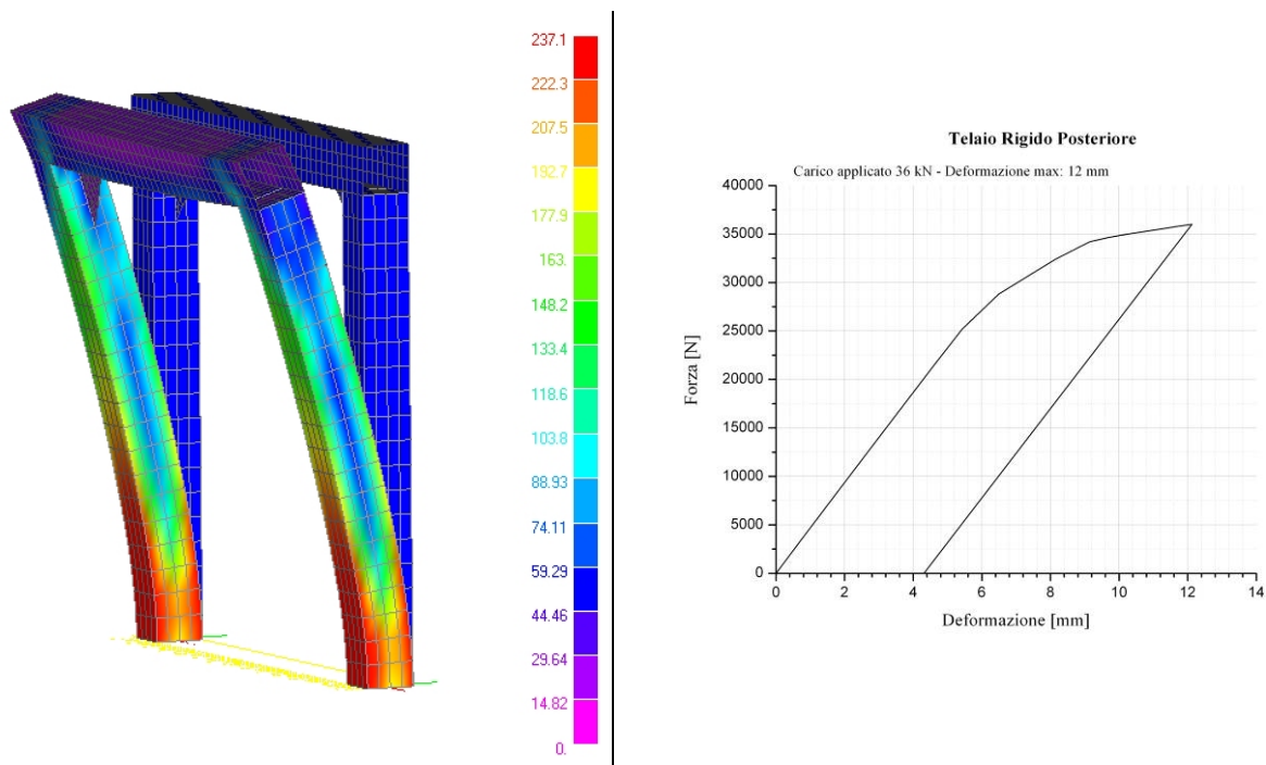
Figura 16. Telaio rigido posteriore: diagramma a falsi colori della tensione [MPa] e diagramma Forza vs. Deformazione
