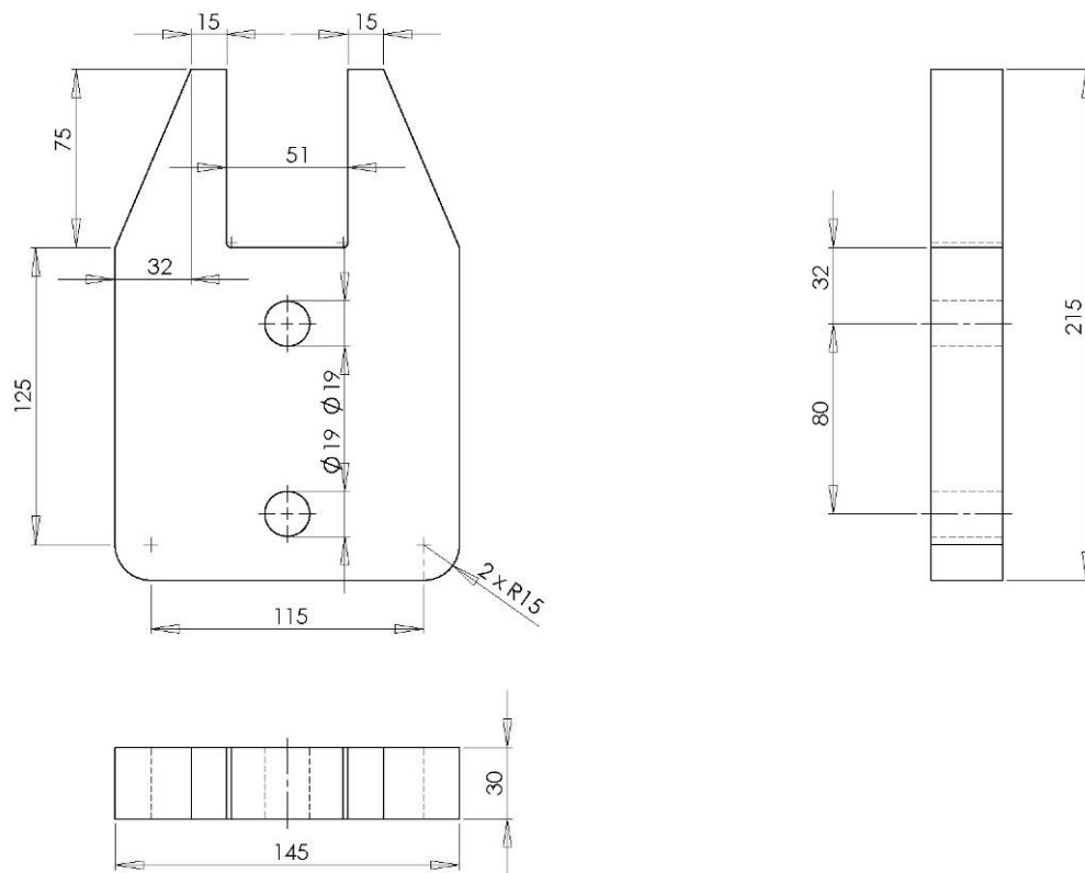
Figura 3. Piastra interna di collegamento per telaio fisso
