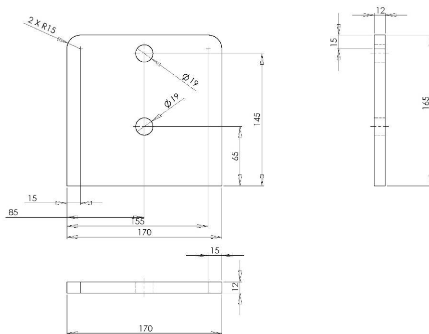
Figura 4. Piastra laterale per telaio fisso
