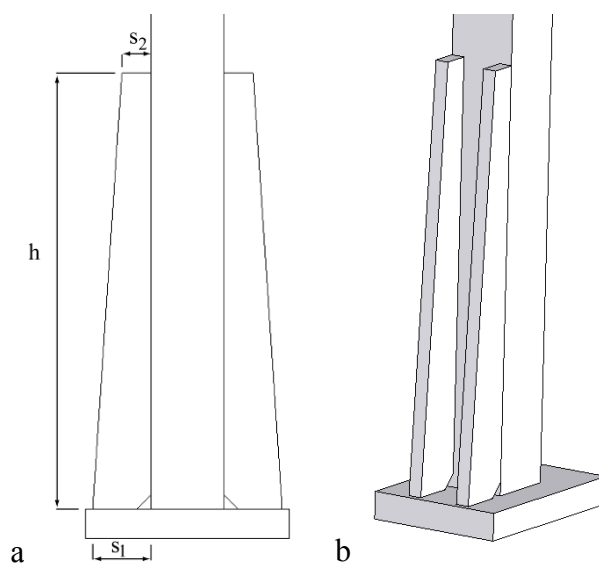
Figura 7. Disposizione flangie di rinforzo
