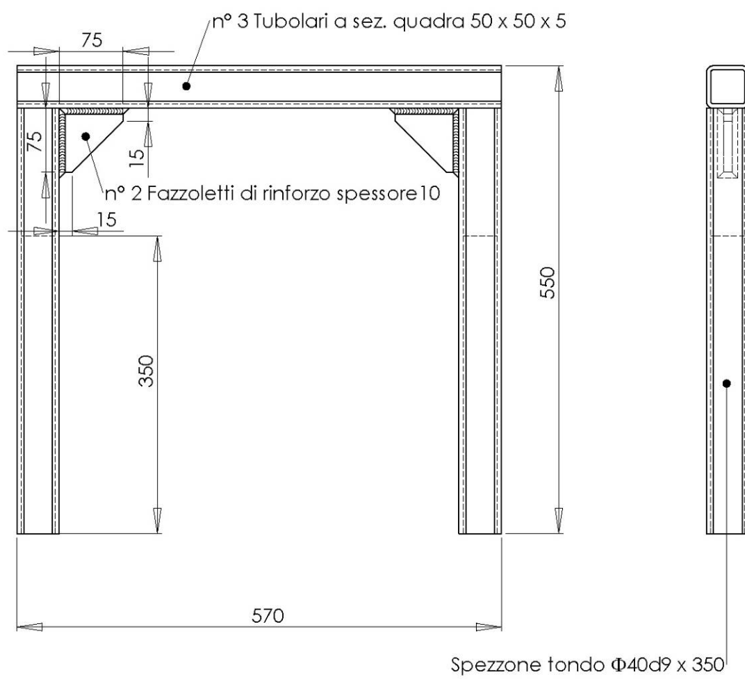
Figura 1. Telaio rigido posteriore
