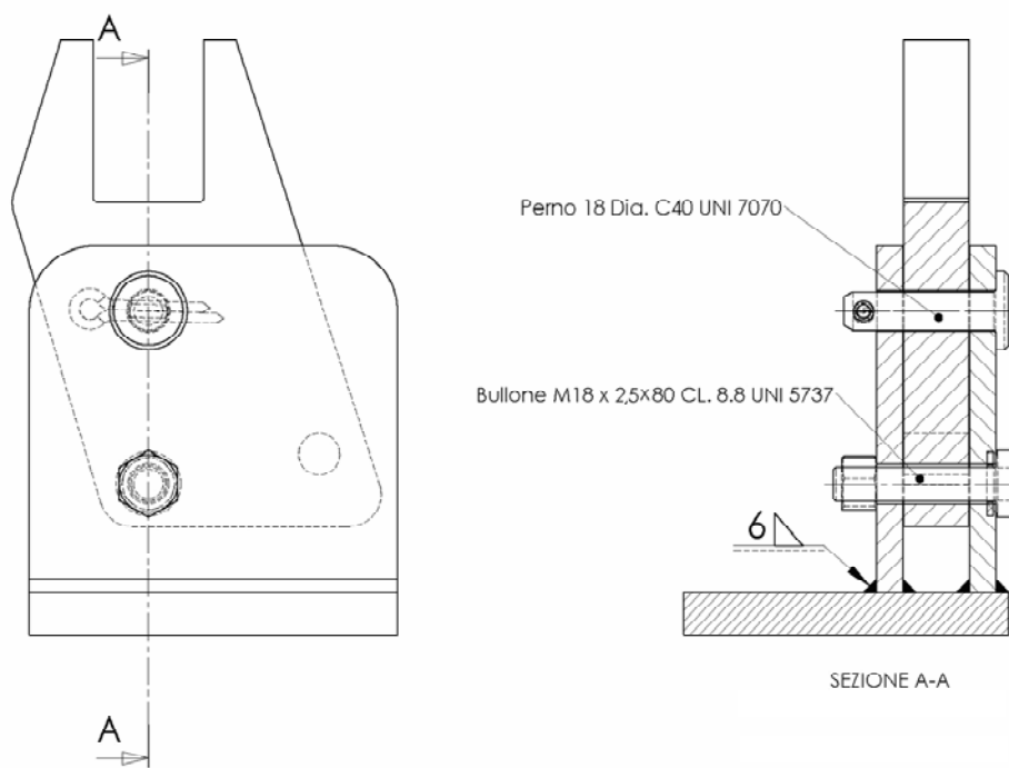
Figura 5. Assieme dell'elemento di collegamento per telaio abbattibile
