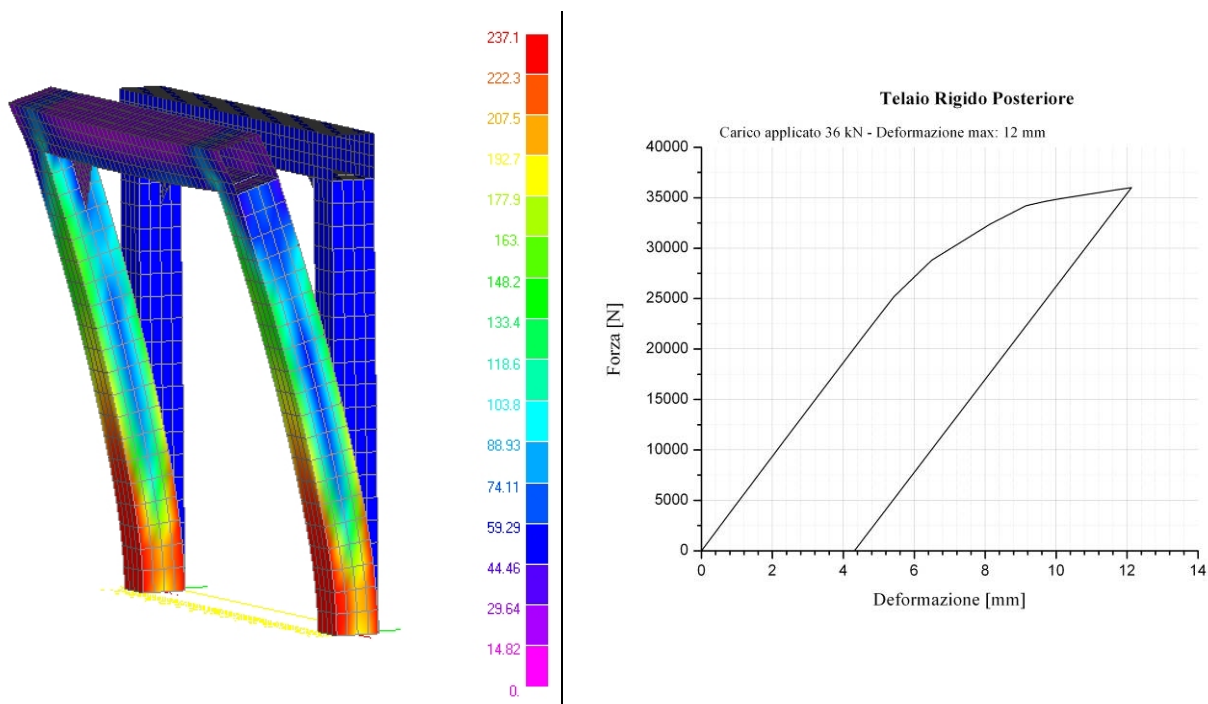
Figura 16. Telaio rigido posteriore: diagramma a falsi colori della tensione [MPa] e diagramma Forza vs. Deformazione
