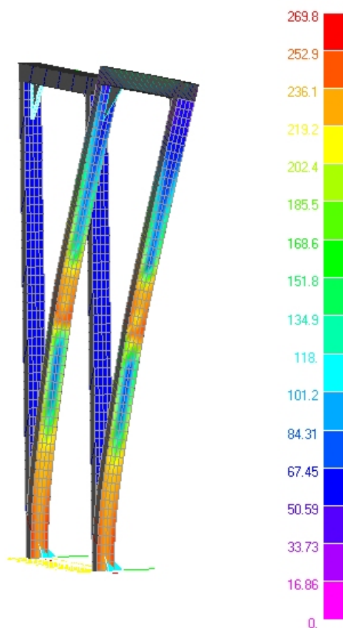
Figura 11. Carico frontale: diagramma a falsi colori della tensione [MPa]
