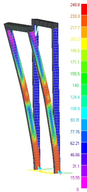
Figura 9. Carico posteriore: diagramma a falsi colori della tensione [MPa]
