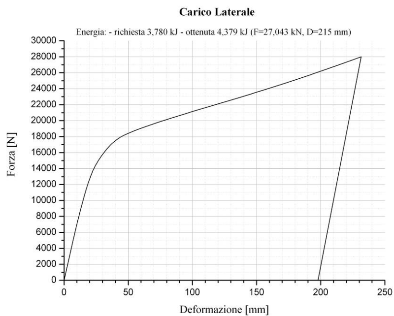
Figura 14. Carico laterale: diagramma Forza vs. Deformazione
