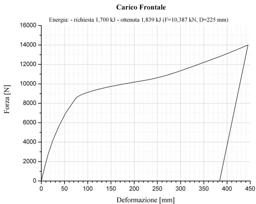
Figura 12. Carico frontale: diagramma Forza vs. Deformazione
