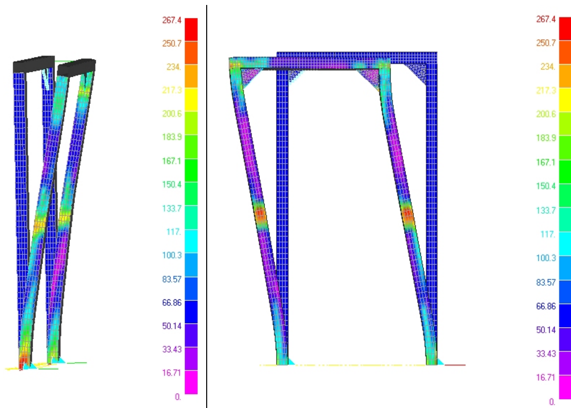
Figura 15. Deformazione residua: diagramma a falsi colori della tensione [MPa]
