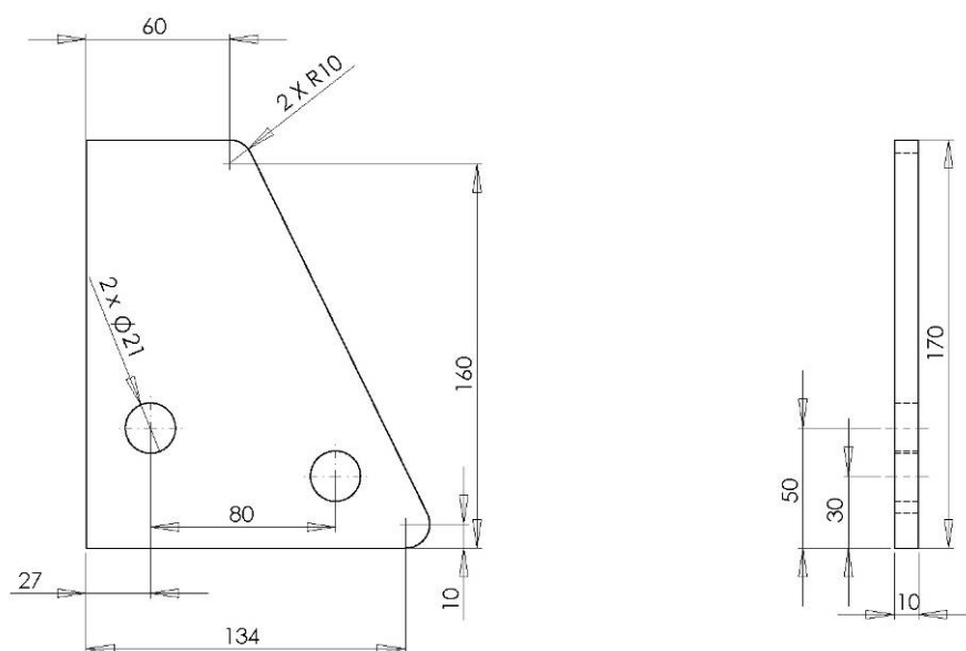
Figura 4. Piastra laterale
