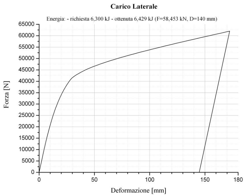
Figura 11. Carico laterale: diagramma Forza vs. Deformazione
