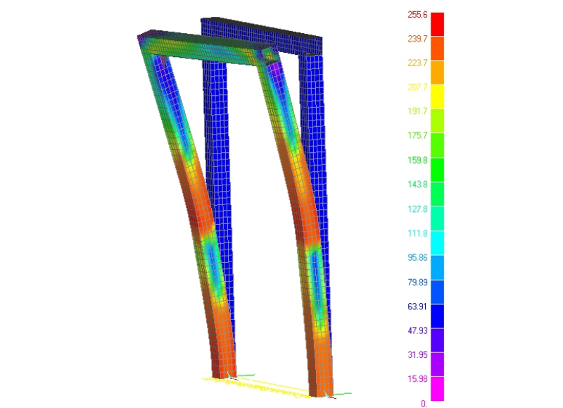
Figura 8. Carico posteriore: diagramma a falsi colori della tensione [MPa]
