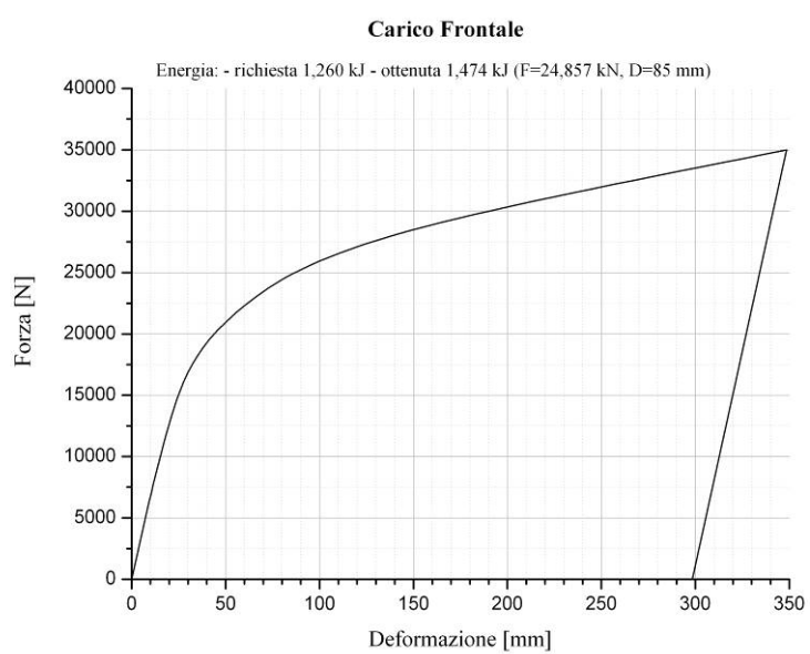
Figura 13. Carico frontale: diagramma Forza vs. Deformazione
