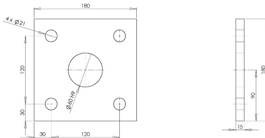
Figura 5. Piastra di base
