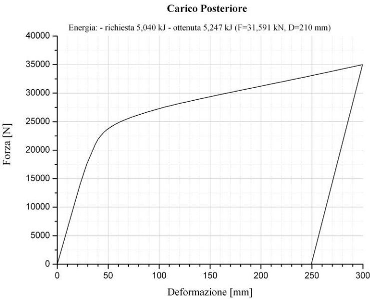
Figura 9. Carico posteriore: diagramma Forza vs. Deformazione
