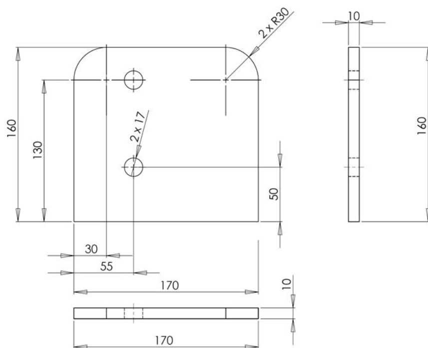
Figura 4. Piastra laterale interna per telaio abbattibile
