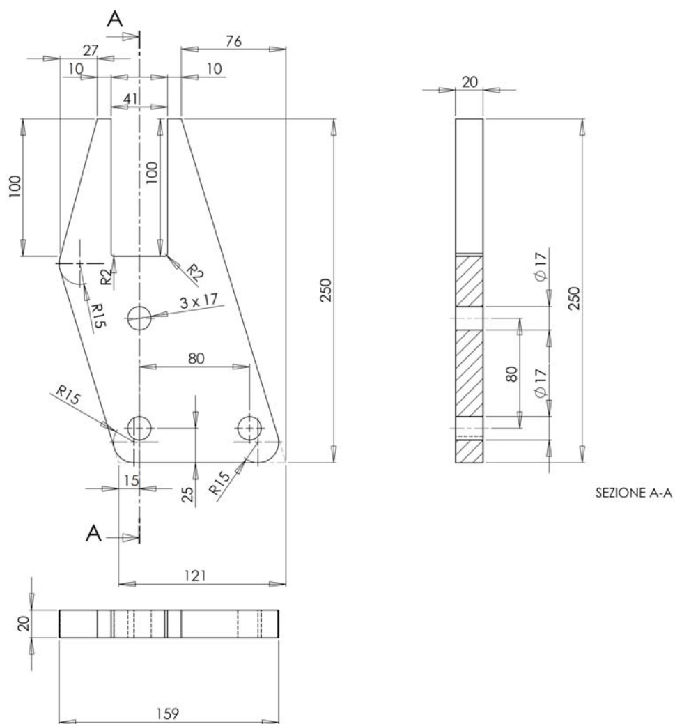
Figura 3. Piastra interna di collegamento per telaio abbattibile
