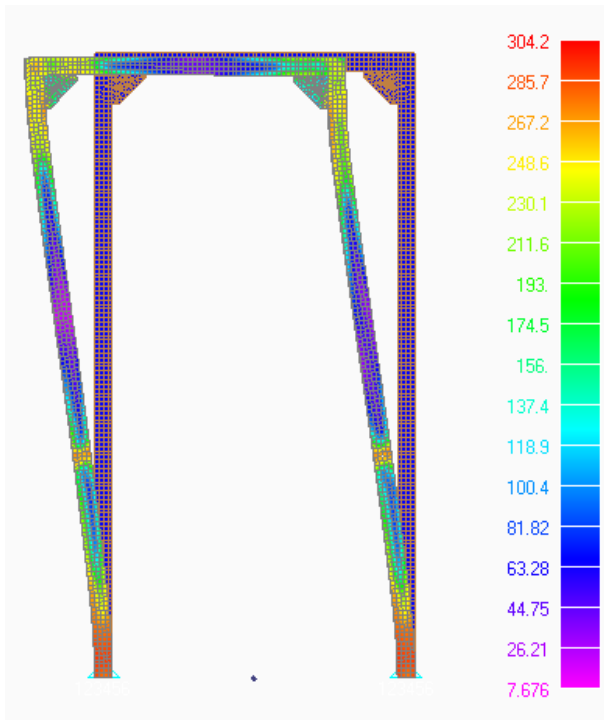
Figura 9. Carico laterale: diagramma a falsi colori della tensione [MPa]
