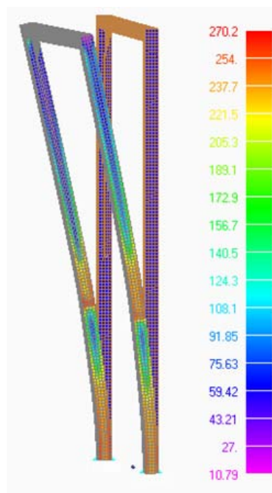
Figura 11. Carico posteriore: diagramma a falsi colori della tensione [MPa]
