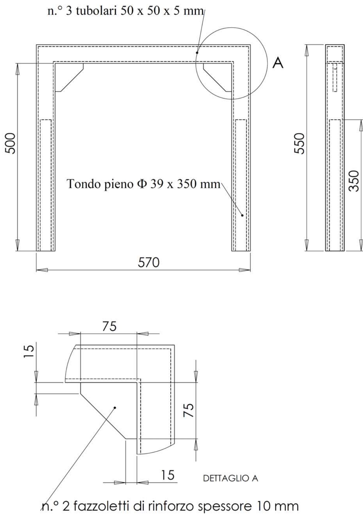
Figura 1. Telaio rigido posteriore
