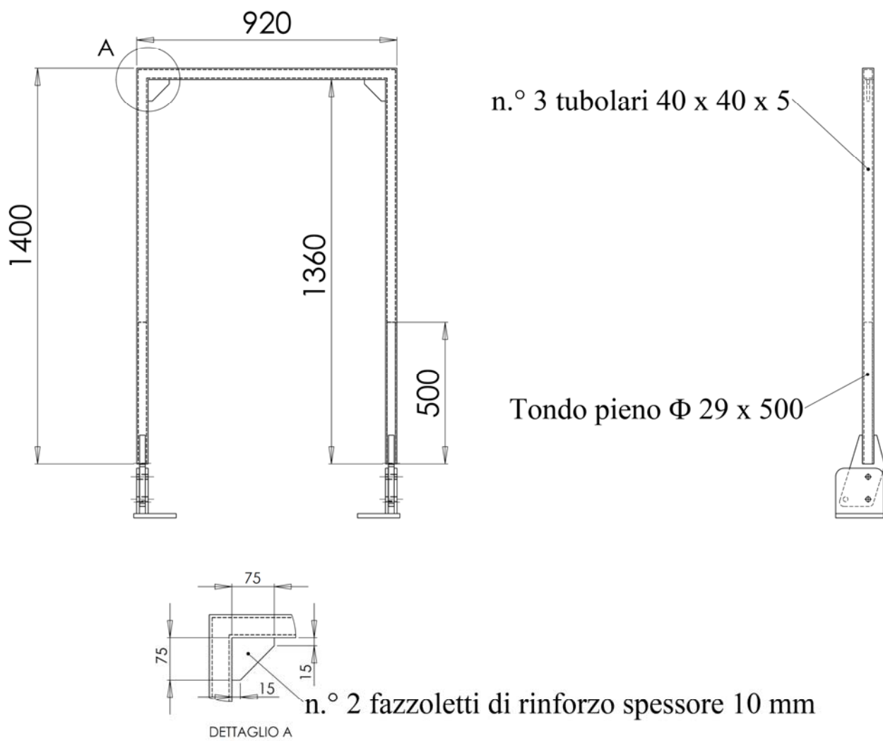
Figura 2. Telaio di protezione anteriore abbattibile
